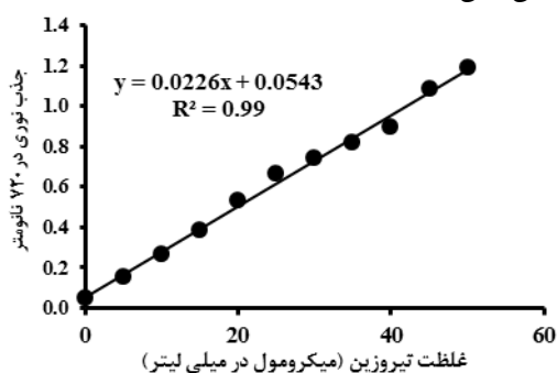
شکل ۲: منحنی استاندارد تیروزین. محور X: غلظت تیروزین (µmole.ml -1 ), محور Y: جذب نوری
