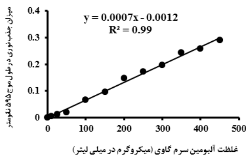
شکل ۱: منحنی استاندارد BSA. محور X: غلظت پروتئین BSA (µg ml -1 ), محور Y: جذب نوری
