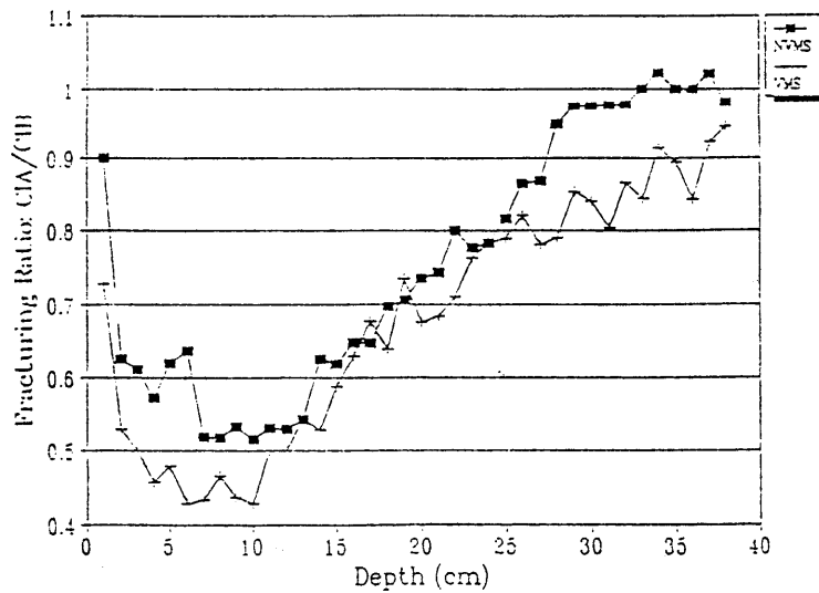
شکل ۶ - بهبود در شاخص مخروطی خاک در اثر زیر شکن زنی با زیر شکن تک شاخه ارتعاشی در دو حالت بدون ارتعاش (NVMS) و ارتعاشی (VMS). CIA به ترتیب مقادیر شاخص مخروطی قبل و بعد از زیر شکن زنی است . نسبتهای کمتر از یک نمایشگر کاهش در مقاومت خاک در اثر زیر شکن زنی می باشد.
