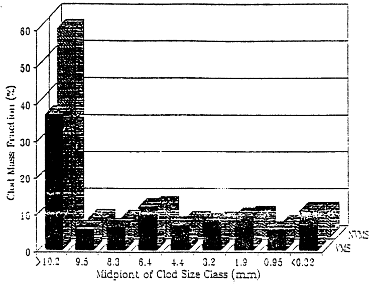
شکل ۷ - نمودار تغییرات ابعاد کلوخه ها بر مبنای وزنی برای زیر شکن تیغه ارتعاشی در دو حالت بدون ارتعاش (NVMS) و ارتعاشی (VMS)
