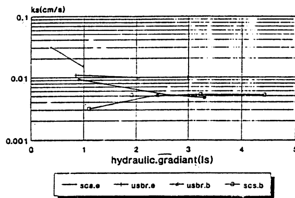
شکل ۱۷- رابطه هدایت هیدرولیکی خاک و گرادیان هیدرولیکی (I) خاکهای مختلف
