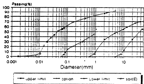
شکل ۸- منحنی های دانه بندی خاک (E) و پوشش ۱۹۸۸ S.C.S
