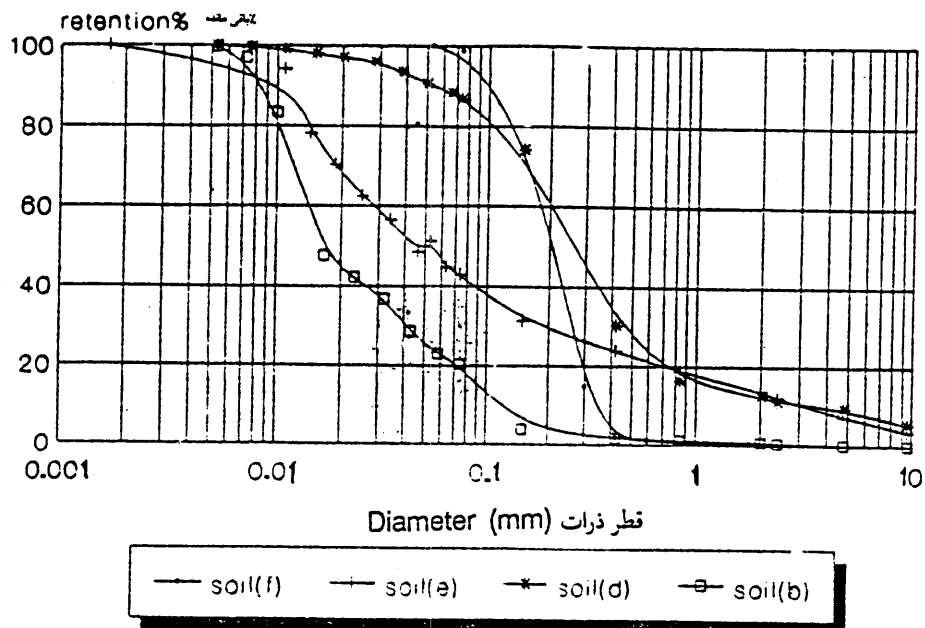
شکل ۲ - منحنی دانه بندی خاک های مورد آزمایش
