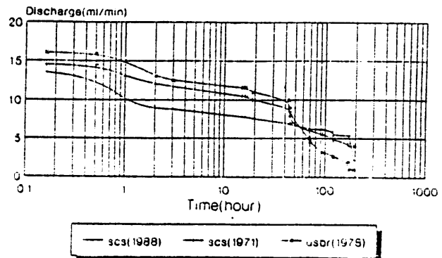
شکل ۱۰- منحنی انسداد پوششها در خاک E
