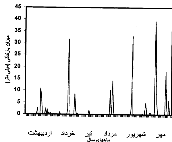
شکل ۳- میزان بارندگی روزانه گرگان در سال ۱۳۷۹
