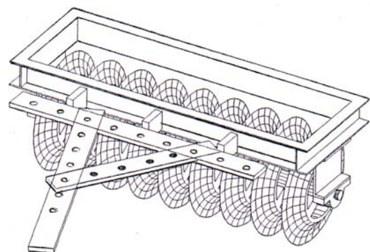
شکل ۱- تصویری شماتیک از غلتک خاک نشان V-شکل
