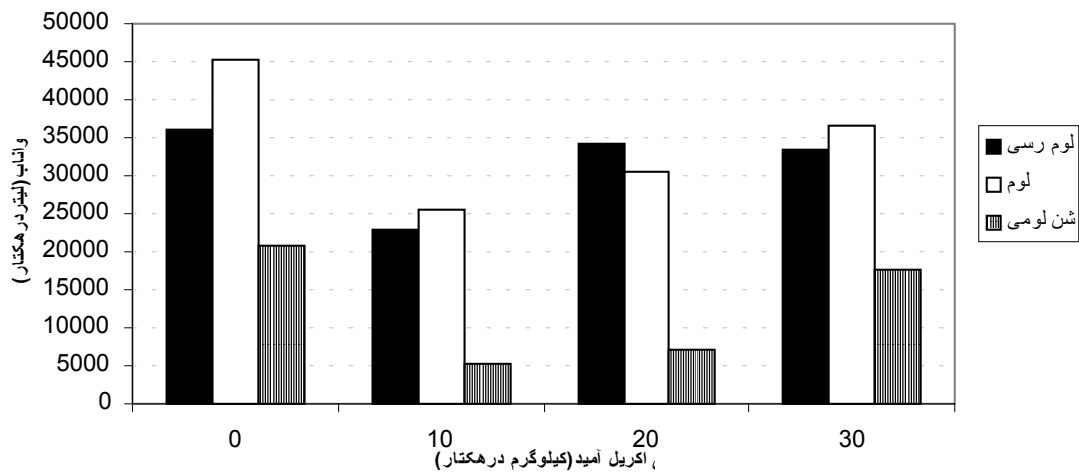
شکل ۴- نمودار رواناب خاکها در تیمارهای مختلف پلی آکریل امید و شدت بارش ۷۹ میلیمتر در ساعت
