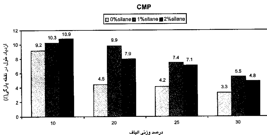
شکل ۹- تغییرات ازدیاد طول در نقطه پارگی بر حسب درصد وزنی الیاف خمیر کاغذ CMP.
