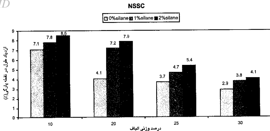
شکل ۸- تغییرات ازدیاد طول در نقطه پارگی بر حسب درصد وزنی الیاف خمیر کاغذ NSSC.
