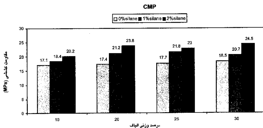
شکل ۳ - تغییرات مقاومت کششی بر حسب درصد وزنی الیاف خمیر کاغذ CMP.
