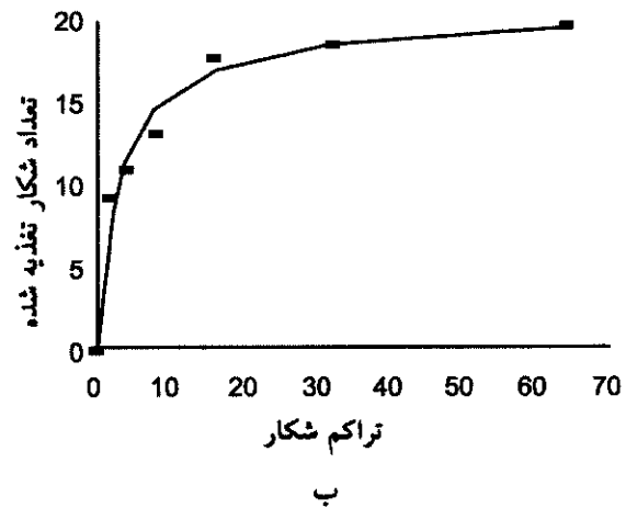
شکل ۱- واکنش تابعی سن شکارگر Andrallus spinidens در تراکم‌های مختلف کرم سبز برگخوار برنج Naranga aenescens الف - پس از ۸ ساعت ب - پس از ۲۴ ساعت
