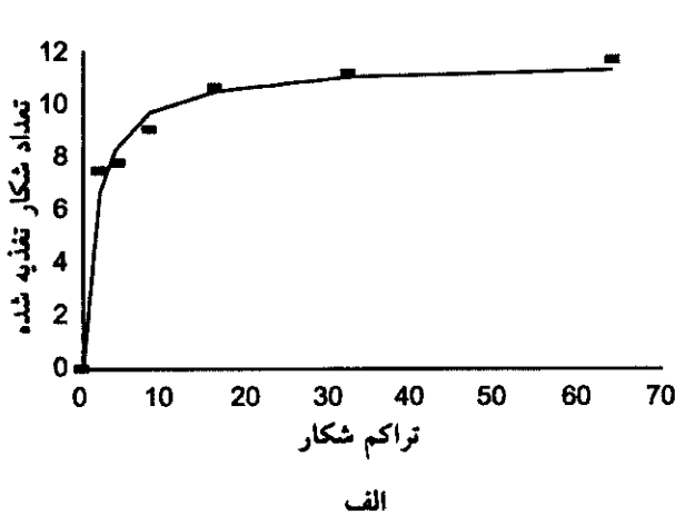
شکل ۱- واکنش تابعی سن شکارگر Andrallus spinidens در تراکم‌های مختلف کرم سبز برگخوار برنج Naranga aenescens الف - پس از ۸ ساعت ب - پس از ۲۴ ساعت
