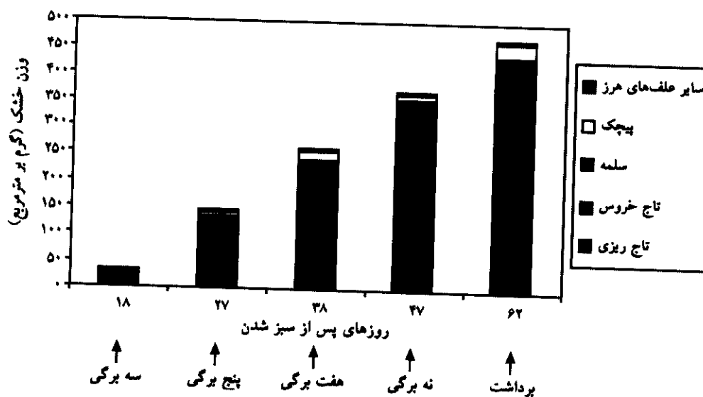
شکل ۲- اثر تیمارهای تداخل ابتدای فصل بر وزن خشک علف‌های هرز به تفکیک گونه آنها.
