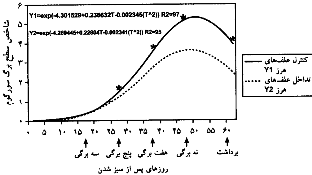
شکل ۵- اثر تیمارهای کنترل و تداخل علف‌های هرز از ابتدای فصل رشد تا مراحل رشدی سورگوم بر شاخص سطح برگ.
