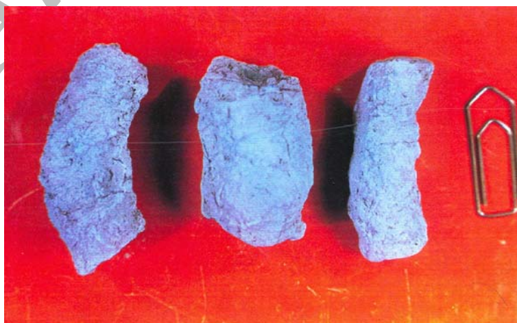
شکل ۱- اشکال کروتویناها در اندازه‌های مختلف.
