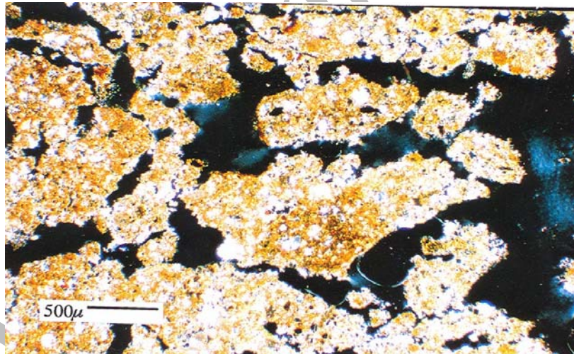
شکل ۴- فابریک داخلی خاکدانه‌ای در کروتوئیناهای افق B_{tb} (تصویر XPL).
