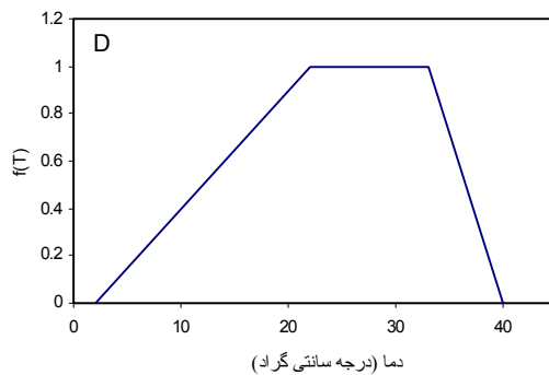
شکل ۱- توابع استفاده شده برای مدل‌سازی واکنش سبزشدن به درجه حرارت شامل: بتا (B)، دو تکه‌ای (S)، درجه دوم (Q)، منحنی (C) و دندان مانند (D).
