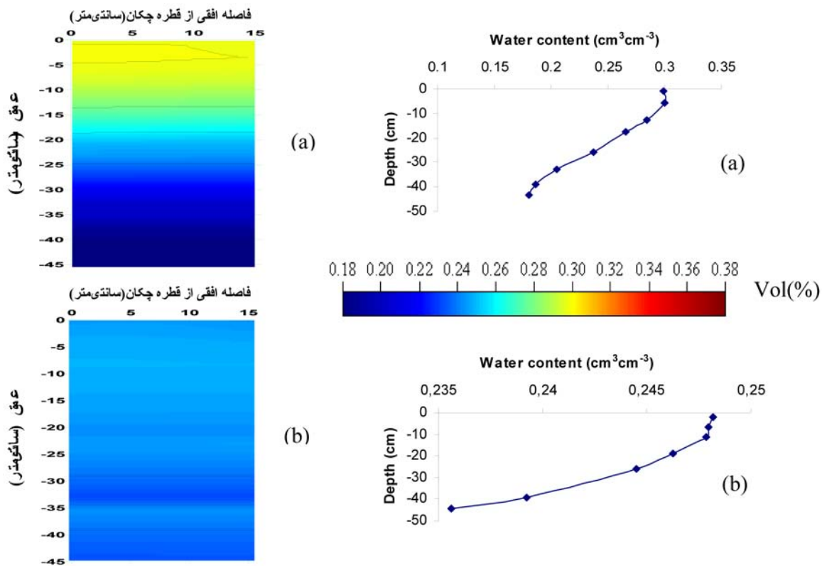
شکل ۶- شبیه‌سازی توزیع رطوبت در خاک الف- ۲ ساعت بعد از آبیاری ب- ۲۴ ساعت بعد از آبیاری.
