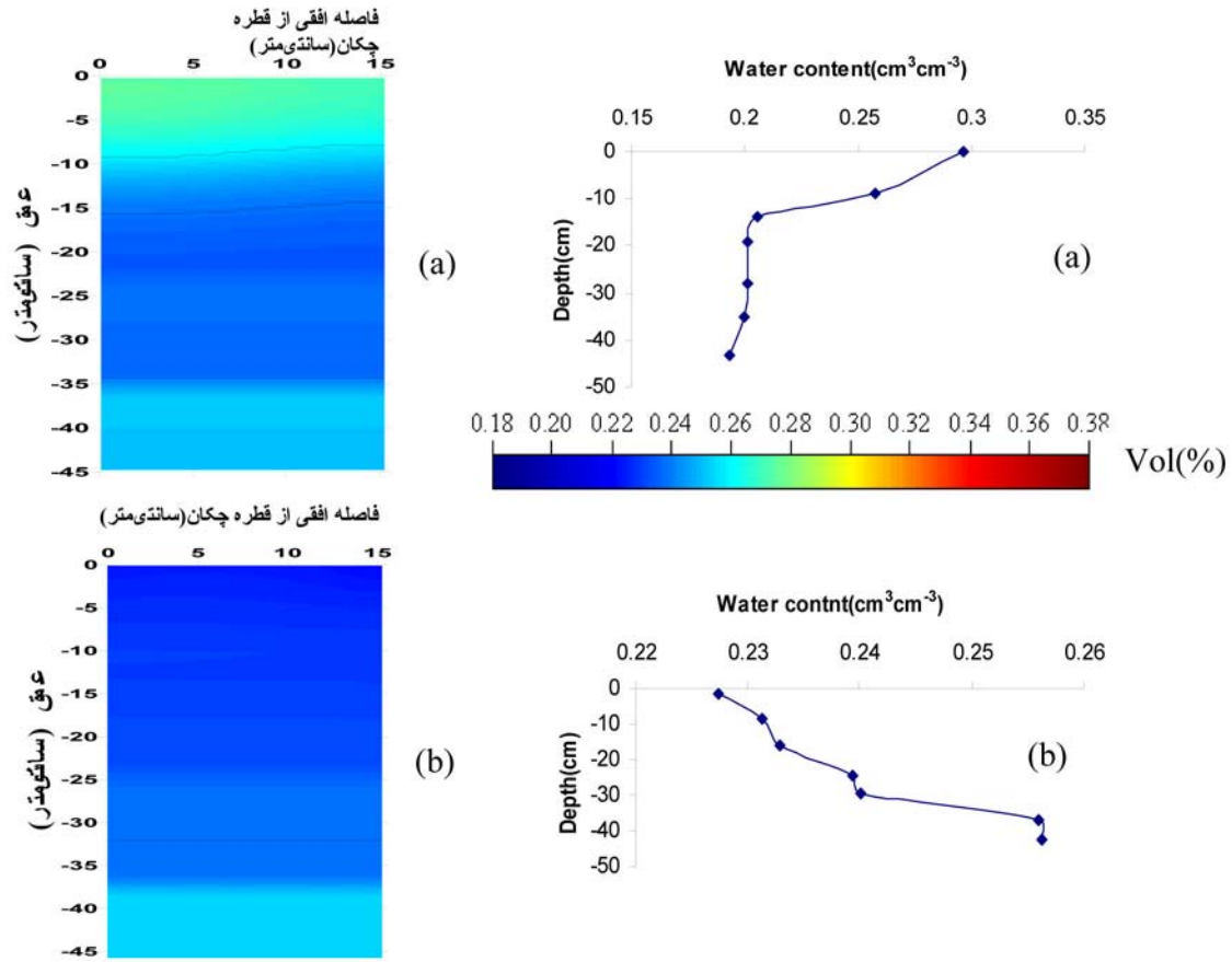
شکل ۸- شبیه‌سازی توزیع رطوبت در خاک الف- ۲ ساعت بعد از دومین آبیاری ب- ۴۸ ساعت بعد از دومین آبیاری.
