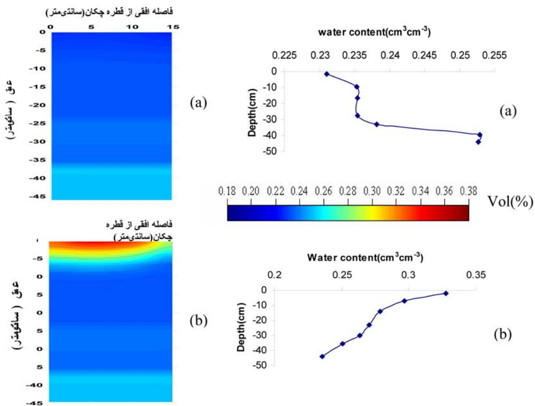
شکل ۷- شبیه‌سازی توزیع رطوبت در خاک الف- ۴۸ ساعت بعد از آبیاری ب- ۳۰ دقیقه بعد از دومین آبیاری.
