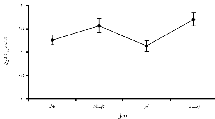
شکل ۴- تغییرات شاخص شانون ( \pm انحراف معیار) برای ماهیان ساحلی تالاب گمیشان (۸۶-۱۳۸۵).
