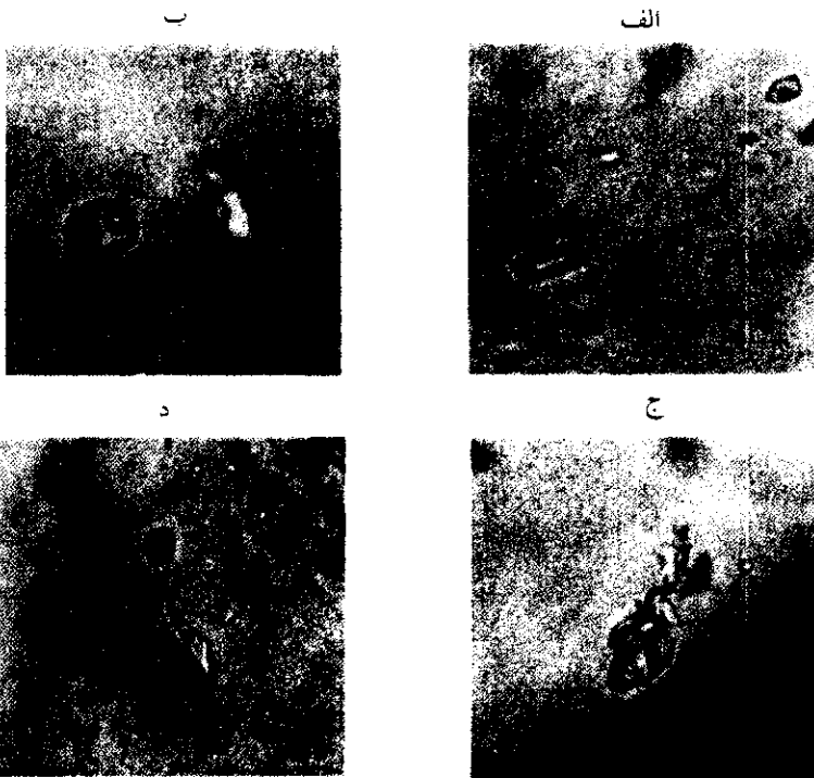
شکل ۶- آنکلوژیونهای اولیه تپیک با ترکیب متفاوت در نمونه‌های مورد مطالعه
