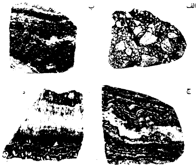
شکل ۱- انواع یافته‌های کانسار کوارتز - اسپیکولاریت (هماتیت)
