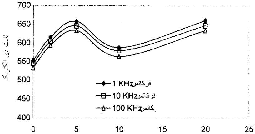
شکل ۵ تغییرات ثابت دی الکتریک بر حسب درصد افزودنی.
