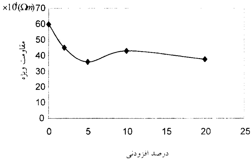
شکل ۶ تغییرات مقاومت ویژه بر حسب افزودنی اکسید نیکل در بسامد ۱۰ kHz.
