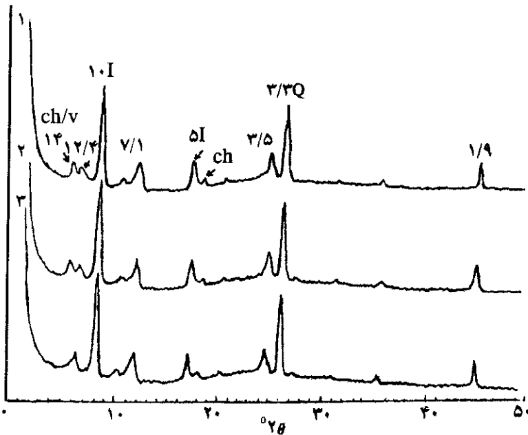
شکل ۳ پراش نگاشت پرتو ایکس از ذرات رس سنگ فیلات هوازده (نیمرخ خاک ۱) پراش نگاشت ۱: نمونه اشباع شده با منیزیم. پراش نگاشت ۲: نمونه ۱ + گلیکول. پراش نگاشت ۳: نمونه اشباع با پتاسیم + دمای 550^{\circ}\text{C} به مدت ۲ ساعت.
