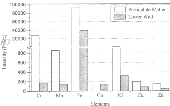
شکل ۴ مقایسه عناصر موجود در دوده خروجی با مواد موجود در جدارة دودکش.
