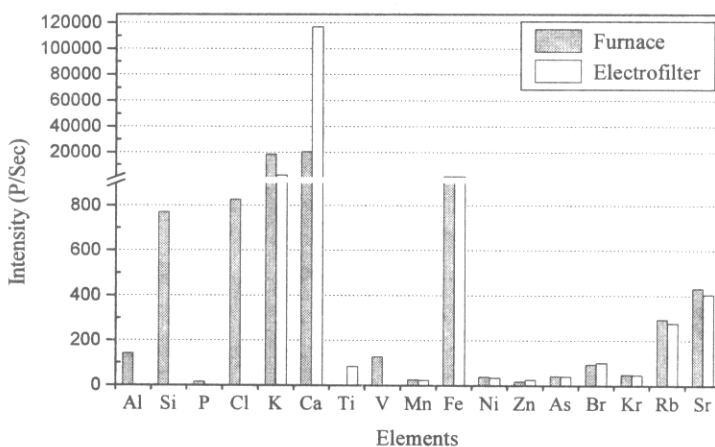
شکل ۲ مقایسه عناصر خروجی از الکتروفیلتر کوره ۳ با مواد داخل کوره.
