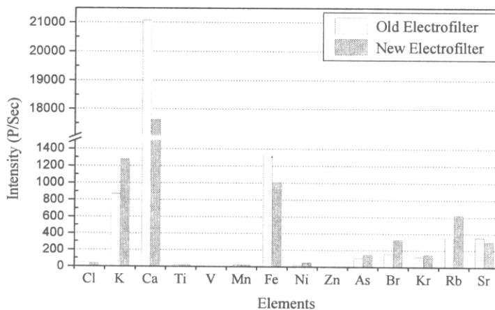
شکل ۳ مقایسه خروجی الکتروفیلتر جدید و قدیم کوره ۲.
