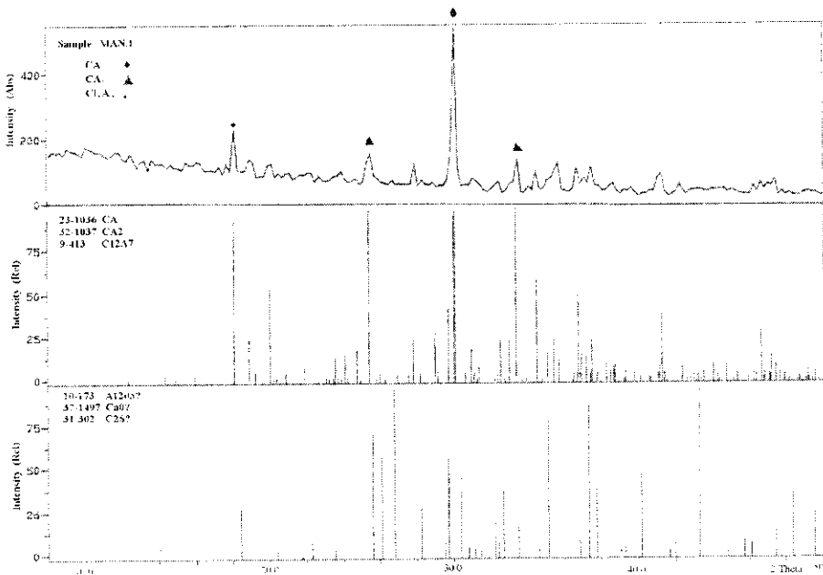
شکل ۲ طرح پراش پرتو X از نخستین نمونه پخت شده در کوره دوار پس از نیم ساعت گرمادهی در
