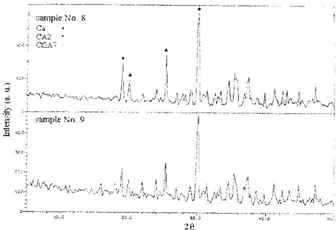
شکل ۳ الگوی پراش نمونه‌های گرمادهی شده در دمای 1550^{\circ}\text{C} به مدت ۳۰ و ۶۰ دقیقه. SID.ir
