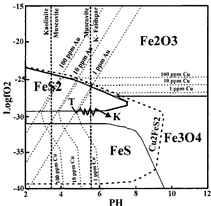
شکل ۱۶ نمودار \text{pH} - \log f\text{O}_2 در دمای T = 350^\circ\text{C} و سایر شرایطی که در نمودار مشخص شده است. مسیر مناسب TK برای کانسار تک I با توجه به پارائزته کانیها مشخص شده است که مسیری نسبتاً اکسیدان است [۱۱].
