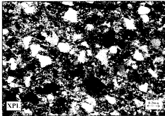
شکل ۲ تصویر میکروسکوپی از سرسیت شیست های سازند تکنار.
