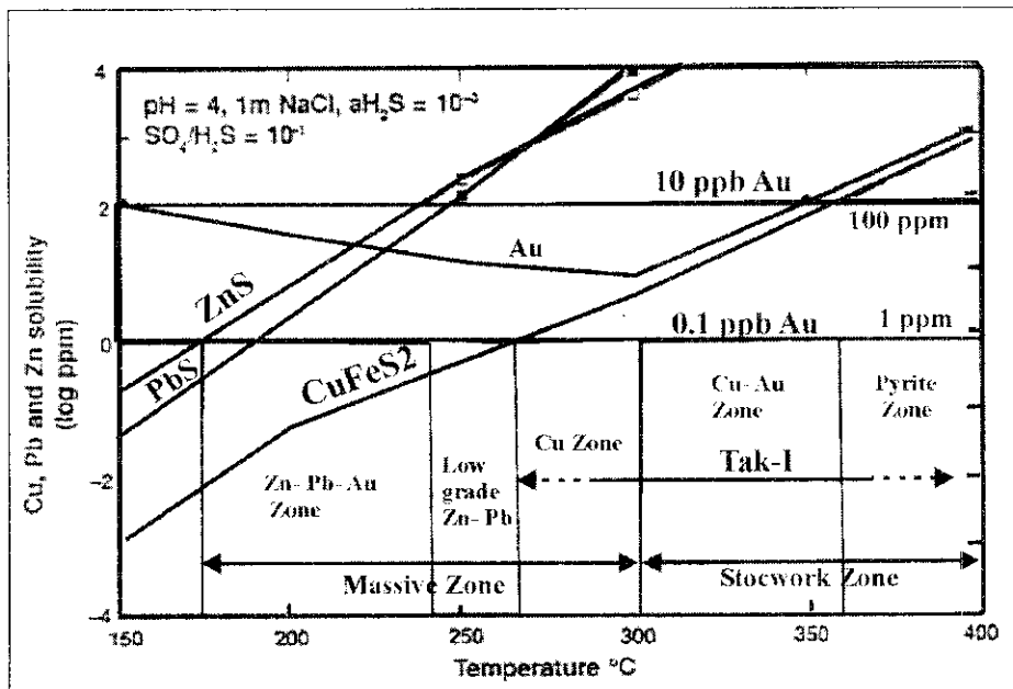
شکل ۱۵ نمودار بررسی وضعیت پایداری و نحوه ناپایدار شدن کمپلکس \text{Cu} ، \text{Au} ، \text{Pb} و \text{Zn} در شرایط \text{pH} = 4 و سایر موارد مشخص شده در شکل ۱۱. محدوده دمایی بخش داربستی و توده‌ای در کانسار ماسیوسولفید تک I ارائه شده است [۱۱].
