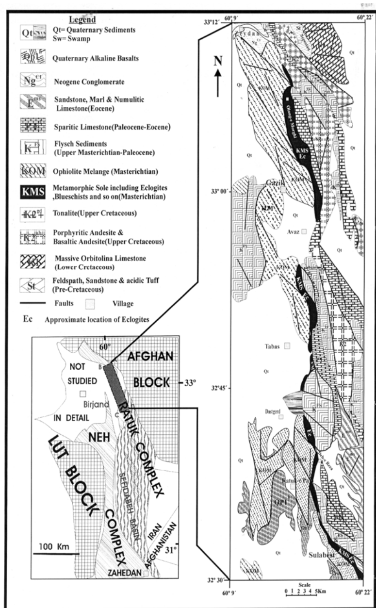
شکل 1 نقشه زمین‌شناسی ساده شده‌ای از منطقه مورد مطالعه و موقعیت منطقه مورد مطالعه در زون جوش خورده سیستان که با چهارضلعی ABCD مشخص شده است (زون جوش خورده سیستان: اقتباس از تیرو و همکاران [3] که مجدداً رسم شده است).
