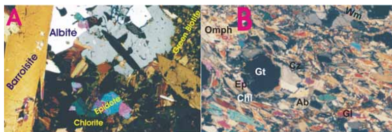
شکل 3 (A) بیوتیت سبز، آلبیت، اپیدوت و بلور کشیده زیبای بارونیزیت در تصویر میکروسکوپی اپیدوت آمفیبولیت سولاست (XPL, 25X). (B) بافت پورفیروبلاستیکی و حضور گارنت و امفاسیت در اکلوزیت دارای شیستوزیه دمدمه (XPL, 20X).
