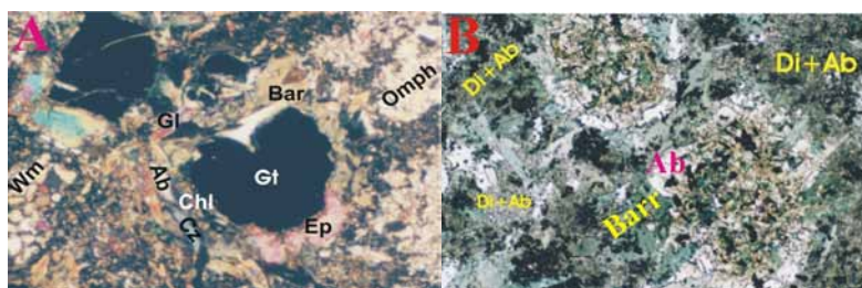
شکل 2 (A) گارنت و امفاسیت (مجموعه کانیایی اولیه رخساره اکلوزیت) و نیز آمفیبول، کلریت، آلبیت و اپیدوت در حاشیه گارنت‌ها که نشانه دگرگونی پسروده اکلوزیت توده ای سولاست به رخساره آمفیبولیت است (XPL, 80X). (B) رشد درهم دیوپسید و آلبیت در نقاط به رنگ سبز خاکستری (NPL, 40X).
