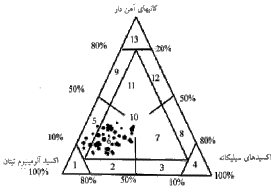
شکل ۸ طبقه بندی انواع بوکسیت بر مبنای نمودار مثلثی کانیهای آهن آلومینیوم و سیلیکاتی (باردوشی ۱۹۸۲) و جایگاه بوکسیت جاجرم در این طبقه بندی.
