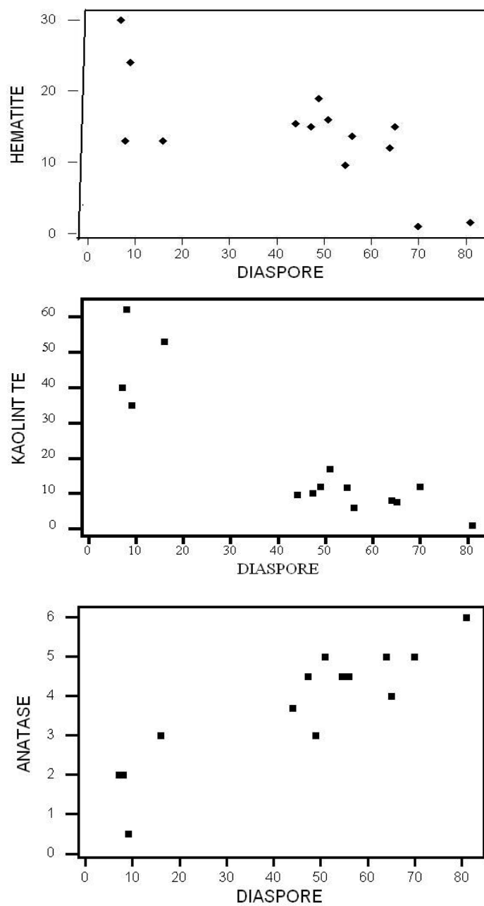
شکل ۷ رابطه بین دیاسپور با کانیهای هماتیت - کائولین و آناتاز.
