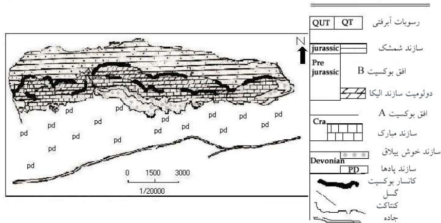
شکل ۲ نقشه زمین‌شناسی محدوده کانسار بوکسیت جاجرم (با تغییراتی بعد از گروه اکتشاف ۱۳۷۰)
