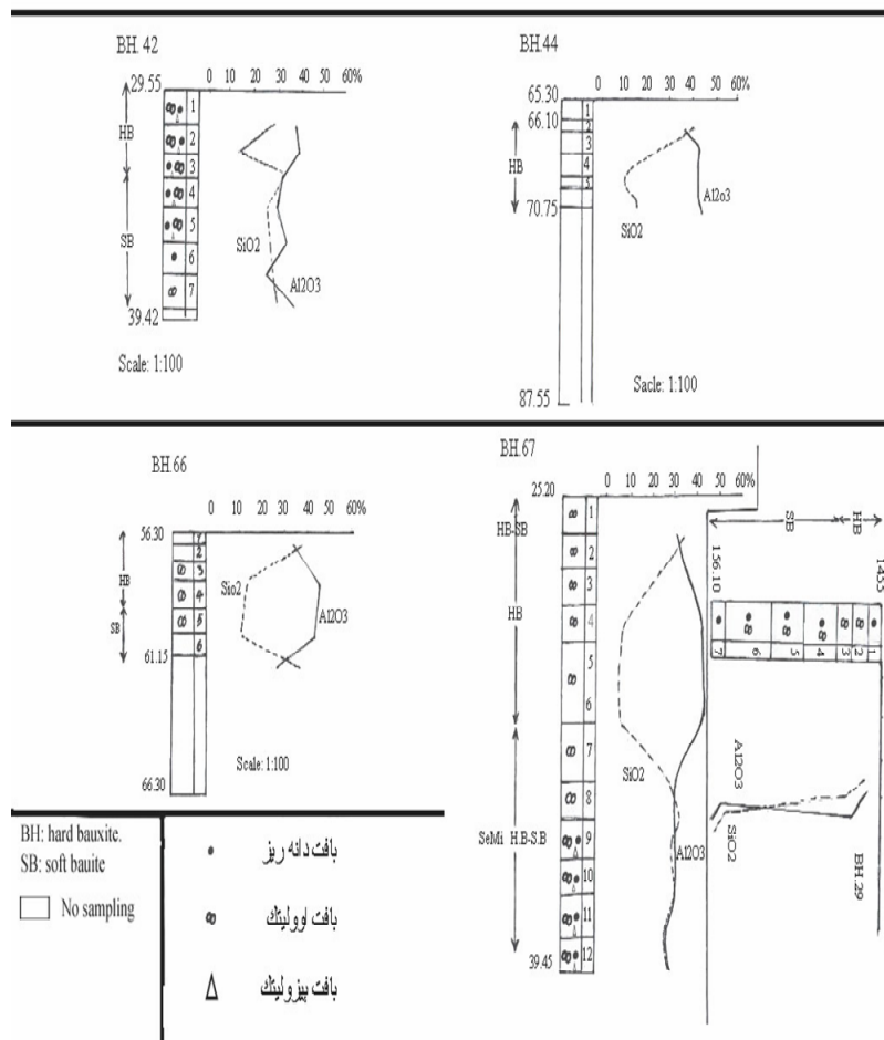
شکل ۶ نمودار خطوط متغیر دیاسپور و کائولین همراه با عمق و نوع بافت در زون ماده معدنی.
