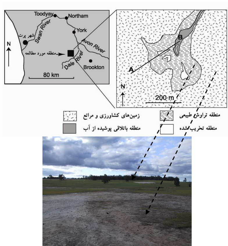
شکل ۲ موقعیت جغرافیای منطقه مورد بررسی در ۱۰۰ کیلومتری شهر پرت در حوزه آبخیز وستدل و پراکندگی عارضه‌های سطحی در توپوسکانس منطقه.
