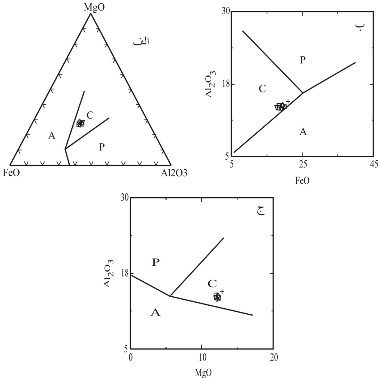
شکل ۴ طبقه بندی محیط زمین ساختی گرانیتوئیدها از روی ترکیب شیمیایی بیوتیت‌ها بر حسب فراوانی الف) \text{FeO}^*\text{-MgO-Al}_2\text{O}_3 (ب) \text{Al}_2\text{O}_3\text{-FeO}^* ج) \text{MgO-Al}_2\text{O}_3 [۱۲]. A: ناکوهزایی آلکان، P: سنگهای پر آلومین و C: سنگهای کالک آلکان است (علائم مورد استفاده مشابه شکل ۲ است).
