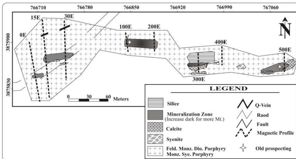
شکل ۳ زمین‌شناسی گستره زون شمال خاوری.
