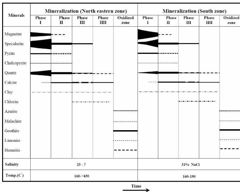
شکل ۴ دنباله پاراژنری زونهای کانی سازی آهن.
