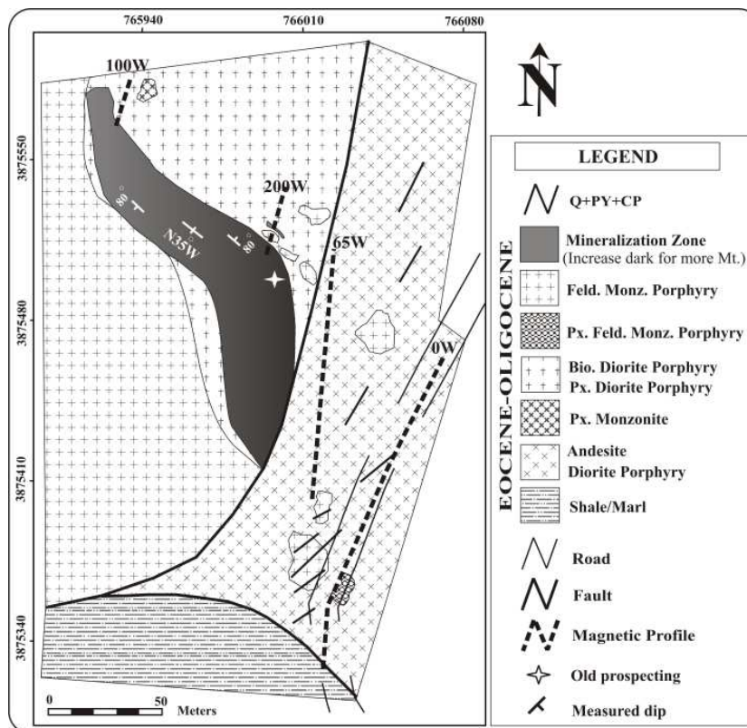
شکل ۲ زمین‌شناسی گستره زون جنوبی.
