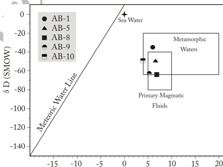
شکل ۳ نمودار مقایسه دامنه تغییرات ایزوتوپ‌های اکسیژن و هیدروژن آب‌های ماگمایی، دگرگونی، گرمایی، اقیانوسی، و سطحی [۲۴].
