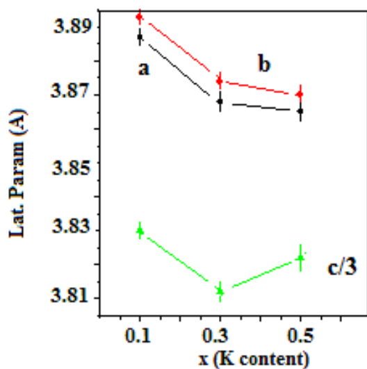
شکل ۴ تغییرات ثابت‌های شبکه‌های a, b, c/3 بر حسب آلایده‌گی پتاسیم.
