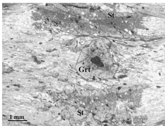
شکل ۵ پورفیروبلاست‌های گارنت (Grt) و استارولیت (St) در زون استارولیت. به شکل‌دار بودن و پایداری این دو کانی توجه کنید.
