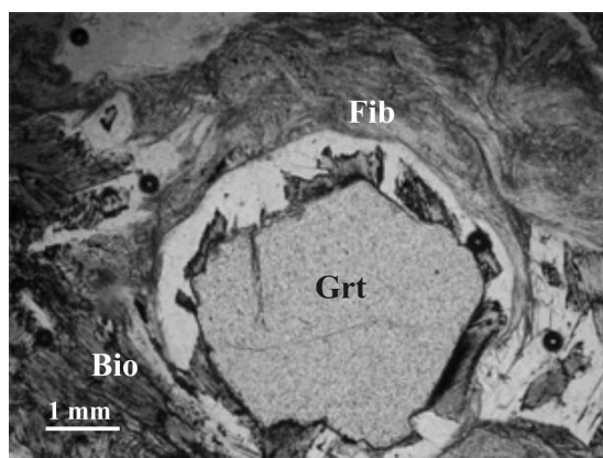
شکل ۹ پورفیروبلاست درشت بلور گارنت در زون گارنت دوم (Grt). به صفحات درشت کانی بیوتیت (Bio) در زمینه و جای‌گزینی بیوتیت با فیبرولیت (Fib) توجه کنید.
