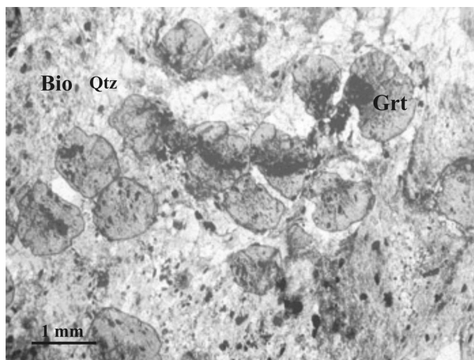
شکل ۳ پورفایروبلاست‌های ریز دانه گارنت (Grt) حاوی ادخال‌های تیره رنگ کانه در یک زمینه و متشکل از بیوتیت (Bio) و کوارتز (Qtz).
