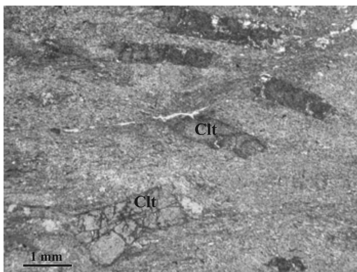
شکل ۲ پورفیروبلاست‌های ماکل‌دار کلریتوئید (Clt).
