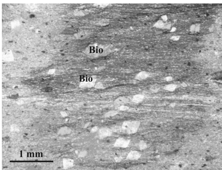
شکل ۱ پورفیروبلاست‌های بیوتیت (Bio) در زون بیوتیت. به چرخش شیستوزیته در پیرامون بیوتیت‌ها توجه کنید.
