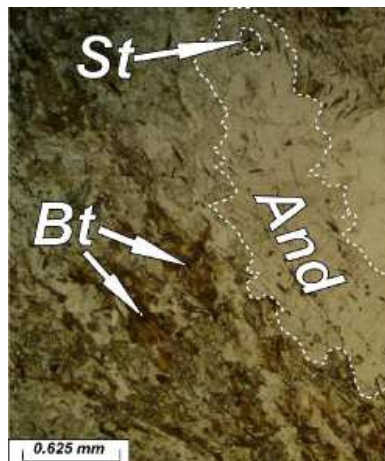
شکل ۸ پورفیروبلست کیاستولیت (And) حاوی ادخال بی‌شکل استارولیت (St) بر گرفته از [۱۳].
