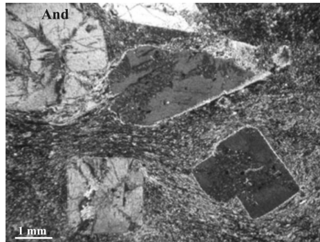
شکل ۷ پورفیروبلست‌های آندالوزیت (And) با ادخال‌های کربن (کیاستولیت). به چرخش شیبستوزیته در پیرامون این پورفیروبلست‌ها توجه کنید.
