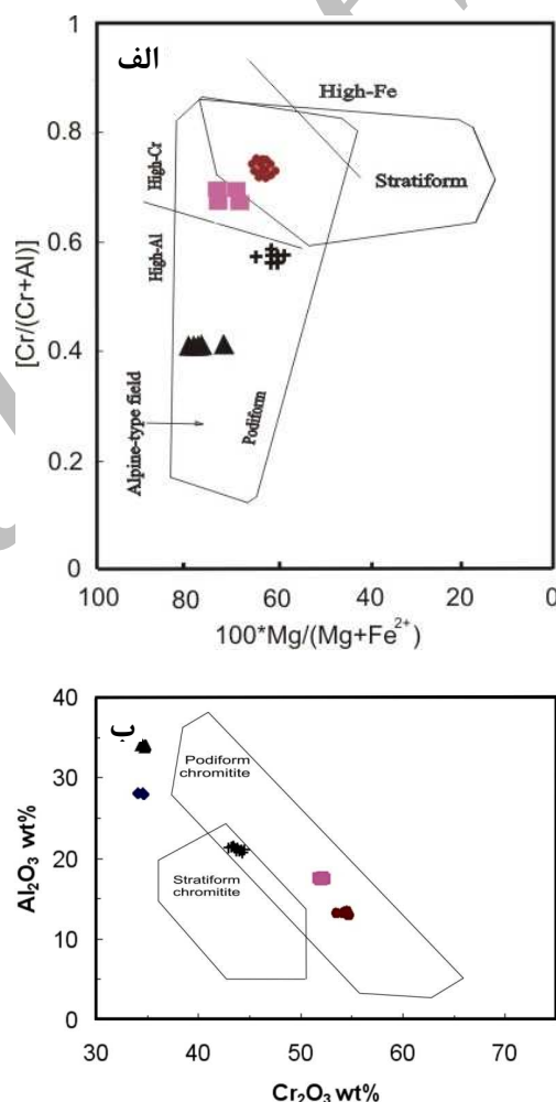
شکل ۵ ترکیب کرومیت‌های افیولیت خوی الف) در نمودار Cr\# نسبت به Mg\# [۱۸] و مقایسه ترکیب کرومیت‌ها با انواع کرومیت‌های Cr ، Al و Fe بالا بر اساس نمودار [۶]، ب) در نمودار Al_2O_3 نسبت به Cr_2O_3 [۱۹]، علائم مشابه شکل ۴ هستند.
