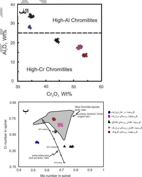
شکل ۴ موقعیت کرومیت‌های مورد بررسی الف) در نمودار Al_2O_3 نسبت به Cr_2O_3 [۱۵]. ب) در نمودار Cr\# نسبت به Mg\# و ارتباط آن با پریدوتیت‌های گوشته‌ای [۱۸].
