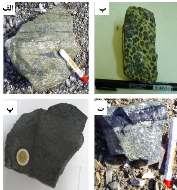
شکل ۲ بافت‌های اولیه در نمونه‌های دستی (الف) بافت افشان (پراکنده) که در بعضی جاها به بافت نواری تبدیل شده است (ب) بافت گرهکی (نودولار) (پ) بافت توده‌ای (متراکم) (ت) بافت نواری در کانسنگ کرومیت و تبدیل لایه‌های کرومیت به لایه‌های سیلیکاتی.
