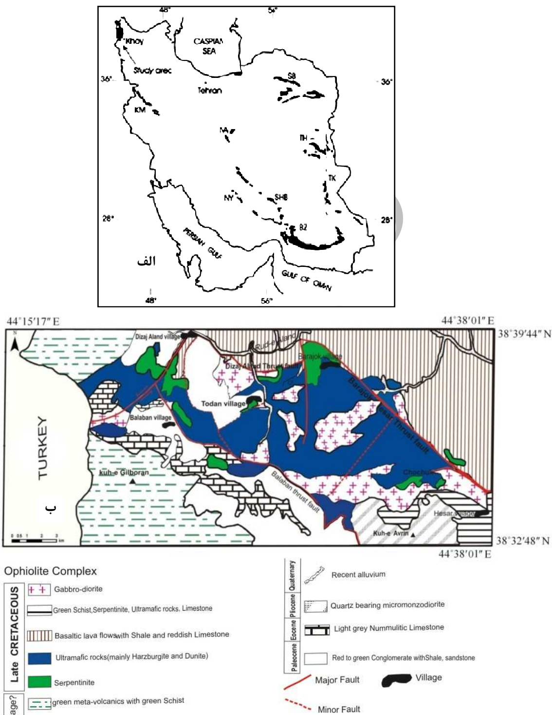
شکل ۱ الف) نقشه پراکندگی افیولیت‌های ایران و موقعیت افیولیت خوی [۱۰۲] ب) نقشه زمین شناسی منطقه مورد بررسی که از کنار هم قراردادن نقشه‌های ۱/۱۰۰۰۰۰ خوی و ۱/۱۰۰۰۰۰ دیزج با تغییرات جزئی تهیه شده است [۱۰، ۹].
