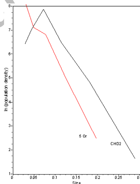
شکل ۶ نمودار CSD فنوکریست‌های کوارتز (5Or, CHD2: اسامی نمونه‌ها).
