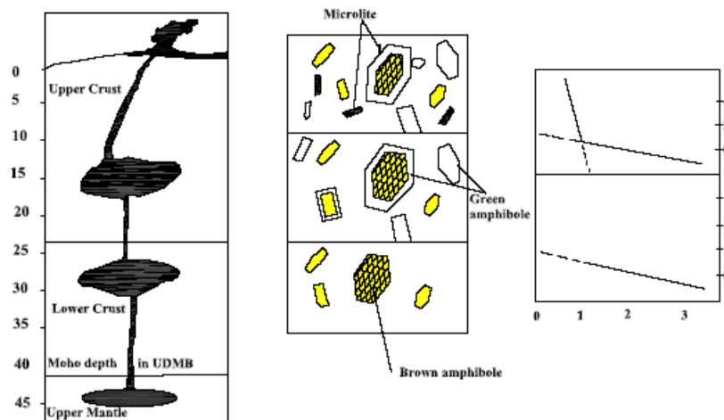
شکل ۱۰ نمودار سرانگشتی نشان دهنده‌ی مکان‌های احتمالی اتاق ماگمایی در یک مقطع عرضی در لیتوسفر، تکامل بافت فنوکریست‌های آمفیبول در طول صعودشان به سطح و الگوی CSD مربوطه در نمونه‌های مورد بررسی در جنوب غرب تهران (عمق موهو در ارومیه دختر از ۱۰). برداشت
