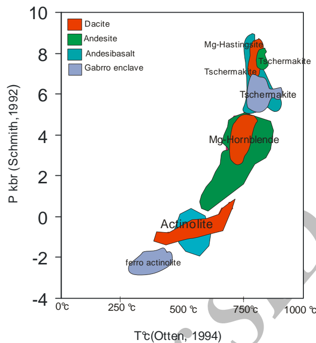
شکل ۹ نمایش دما نسبت به فشار در آمفیبول‌های مورد بررسی.
