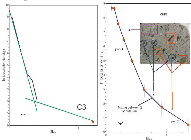
شکل ۸ (الف، ب، پ) چگونگی خمش در نمودارهای وابسته به CSD در فنوکریست‌های آمفیبول مورد بررسی (مقاطع نازک متعدد مورد بررسی با بلورهای آمفیبول بزرگ و کوچک).
