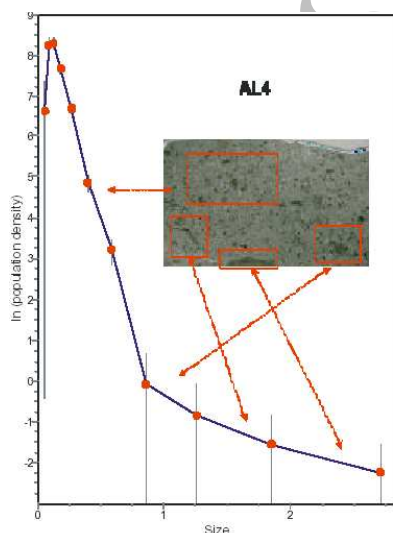
شکل ۷ نمودار CSD فنوکریست‌های آمفیبول در نمونه‌های آندزیتی و داسیت (هریک از منحنی‌ها بررسی CSD را روی یک مقطع نازک جداگانه نشان می‌دهد).
