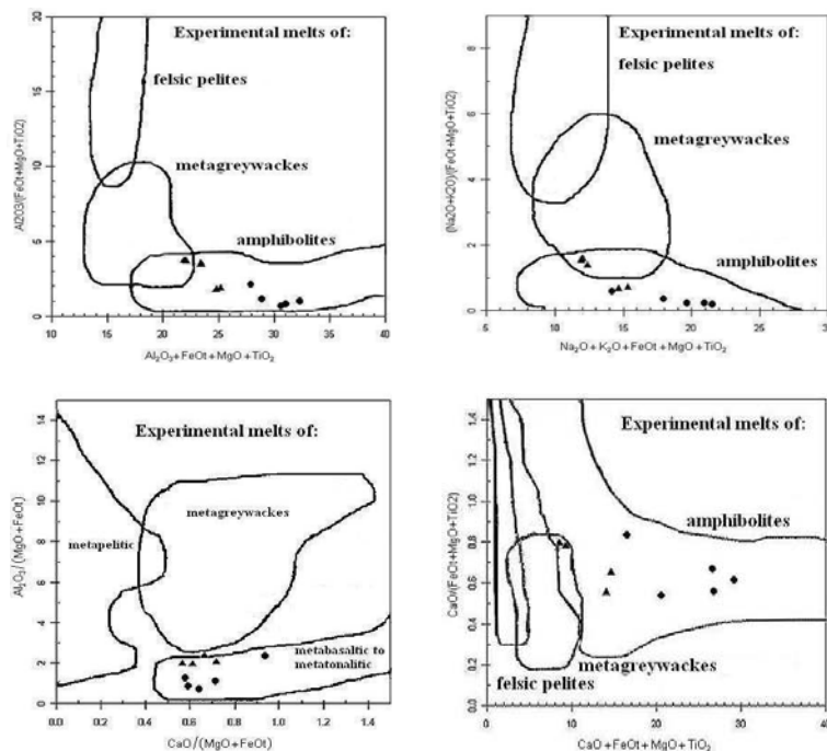
شکل ۱۵ قلمرو ترکیبی گدازه‌های تجربی مشتق از گداخت پلیت‌ها، متاگرایواک‌ها و آمفیبولیت‌ها [۳۱-۳۳] و ترکیب نمونه‌های مافیک منطقه به-عنوان ترکیب ماگمای مادر (علائم مشابه شکل ۷).
