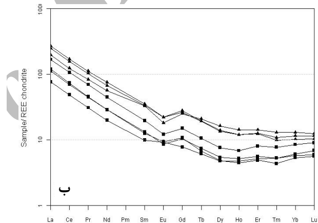
شکل ۱۳ الف) نمودار عنکبوتی عناصر نادر خاکی برای نمونه‌های گرانیتی و گرانودیوریتی منطقه‌ی مورد بررسی بر اساس داده‌های کندریت [۳۷]. ب) نمودار عنکبوتی عناصر نادر خاکی بر اساس داده‌های کندریت [۳۸] ترسیم شده است.
