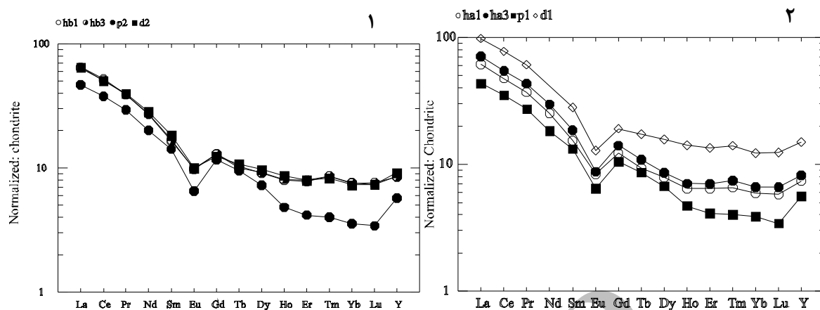
شکل ۷ الف) ۱ و ۲) نمودار عناصر نادر خاکی بهنجار شده نسبت به کندریت در دو نیمرخ مورد بررسی، بیانگر شیب نزولی، تهی شدگی در یوروییوم و کاهش غلظت از LREEs به طرف HREEs
