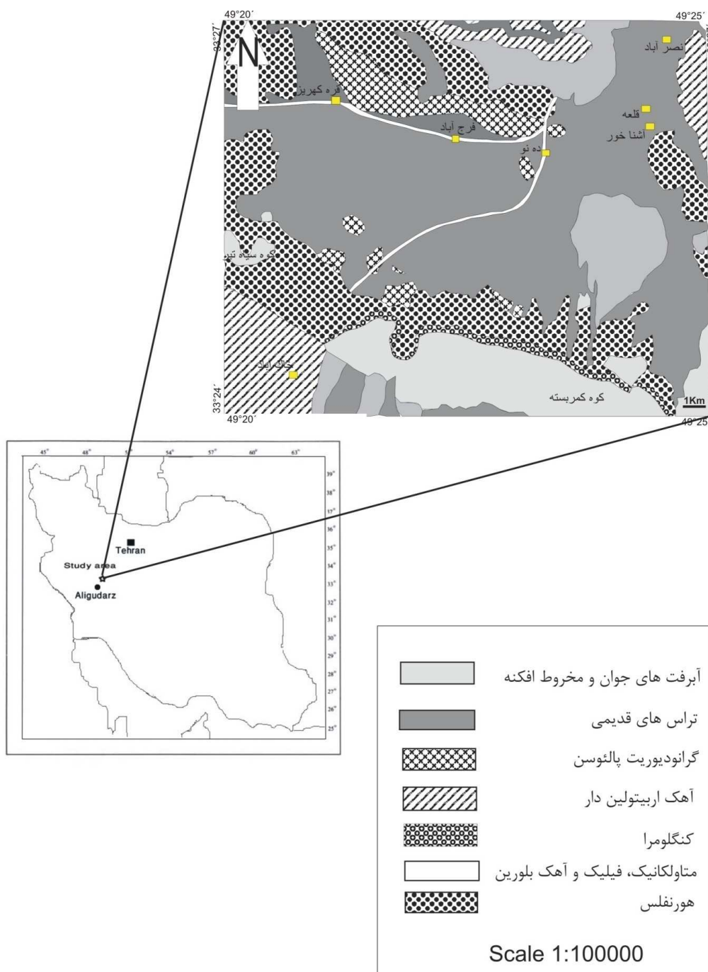
شکل ۱ شمایی از نقشه زمین‌شناسی منطقه مورد بررسی از سهیلی و همکاران (۱۳۷۱) [۵].
