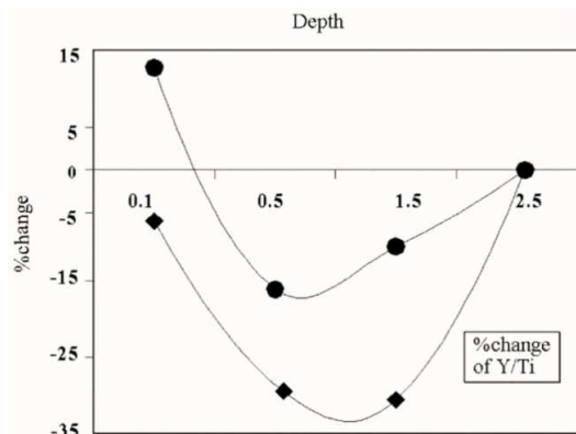
شکل ۶ در صد تغییرات مقادیر عناصر Nb, Ta, Zr, Hf, Y, U نسبت به Ti در نمونه‌های هوازده Ha و Hb در اعماق مختلف در واحد متر.
