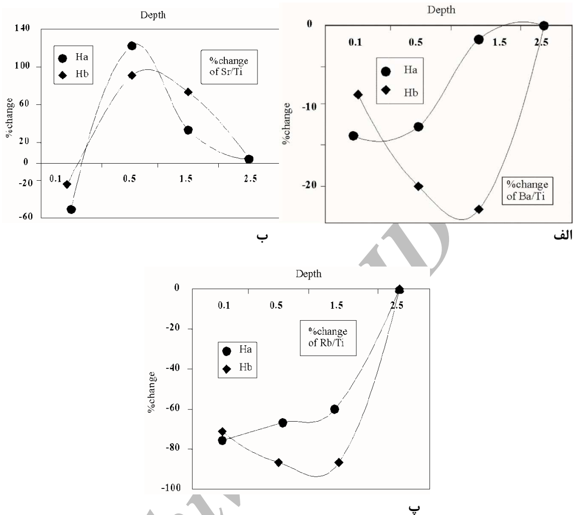
شکل ۵ درصد تغییرات عناصر Sr, Ba, Rb نسبت به Ti در نمونه های هوازده Ha و Hb در اعماق مختلف در واحد متر.
