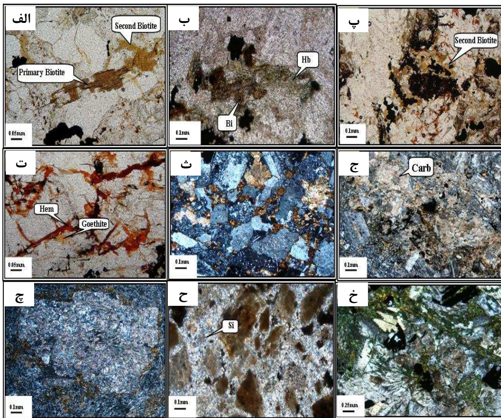
شکل ۵. زون‌های مختلف دگرسانی منطقه‌ی مورد بررسی در مقطع نازک. الف) بیوتیت ثانویه حاصل تبلور مجدد بیوتیت اولیه (نور PPL). ب) بیوتیت ثانویه به صورت جانشینی در هورنبلند (نور PPL). پ) بیوتیت ثانویه به صورت پراکنده در متن سنگ (نور PPL). ت) رگچه‌های اکسید آهن در حال تبدیل به گوتیت در زون دگرسانی پتاسیک (نور PPL). ث) دگرسانی سریسیت + کربنات در سنگ هورنبلند مونزونیت (نور XPL). ج) دگرسانی کربناتی در سنگ هورنبلند دیوریت (نور XPL). چ) تبدیل بلور فلدسپات به کربنات و سریسیت در زون دگرسانی کربنات + سریسیت در سنگ هورنبلند مونزوسینیت پورفیری (نور XPL). ح) دگرسانی سیلیسی در توف (نور XPL). خ) دگرسانی پروپیلیتیک در سنگ مونزوسینیت (نور XPL).
