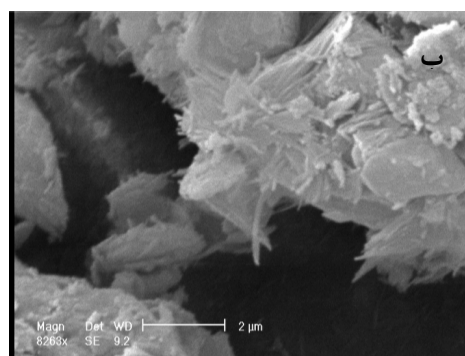
شکل ۵ تصاویر میکروسکوپ الکترونی از بلورهای کلسیت و فیبرهای پالیگورسکایت در کالکریت مورد مطالعه.
