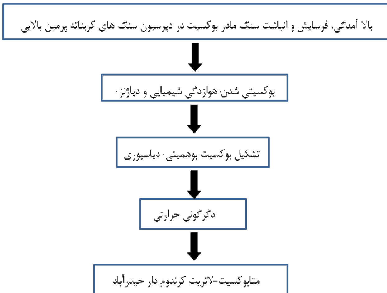
شکل ۸ خلاصه‌ای از فرآیندهای موثر در تشکیل و شکل‌گیری کانسار بوکسیت-لاتریت حیدرآباد به‌صورت شماتیک.
