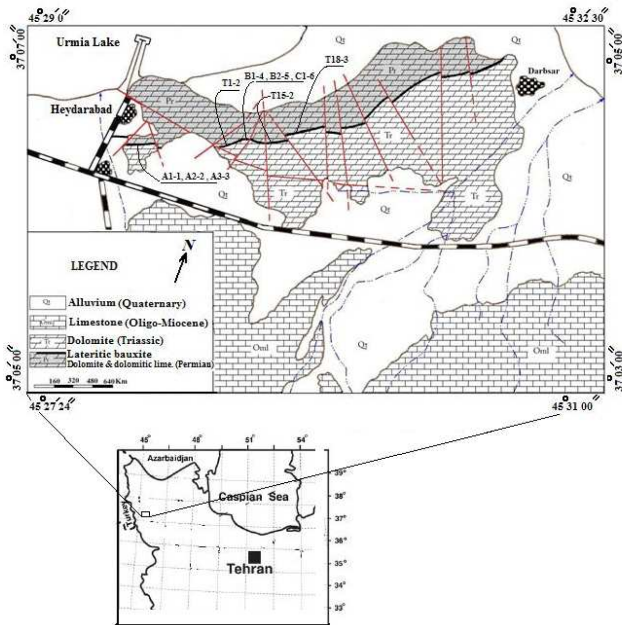
شکل ۱ نقشه زمین‌شناسی ساده شده از کانسار بوکسیت-لاتریت حیدرآباد اقباس از [۸] با تغییرات جزئی، موقعیت نمونه‌های برداشته شده در شکل نشان داده شده است.
