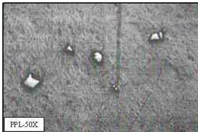
شکل ۲ تصویر میکروسکوپی نور عبوری از بافت انتشاری کانسنگ کرومیت در منطقه چاه‌یابو و چشمه‌پلنگ.
