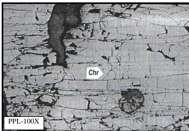
شکل ۱۳ تصویر میکروسکوپی نور بازتابی از بافت میلونیتی تحت تأثیر خردشدگی شدید در مناطق گسلی ایجاد شده است. (Chr = Chromite)
