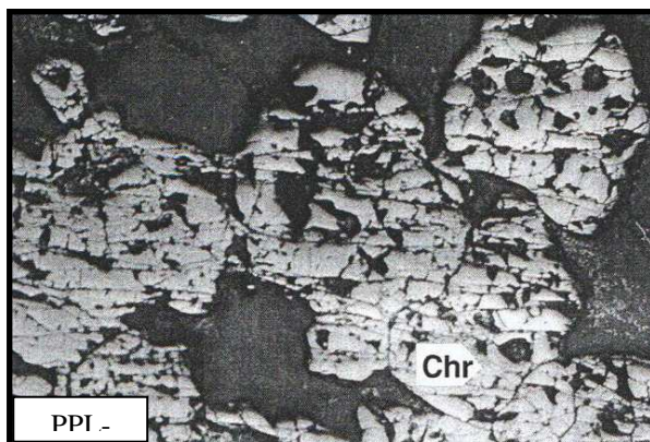
شکل ۷ تصویر میکروسکوپی نور بازتابی دانه‌های بیضی شکل کرومیت در زمینه‌ی سیلیکاتی، منطقه‌ی چشمه‌پلنگ. در این نمونه بافت گره‌ای طی فرایند زمین‌ساختی به بافت کاناکلاستیکی تبدیل شده است. (Chr = Chromite).
