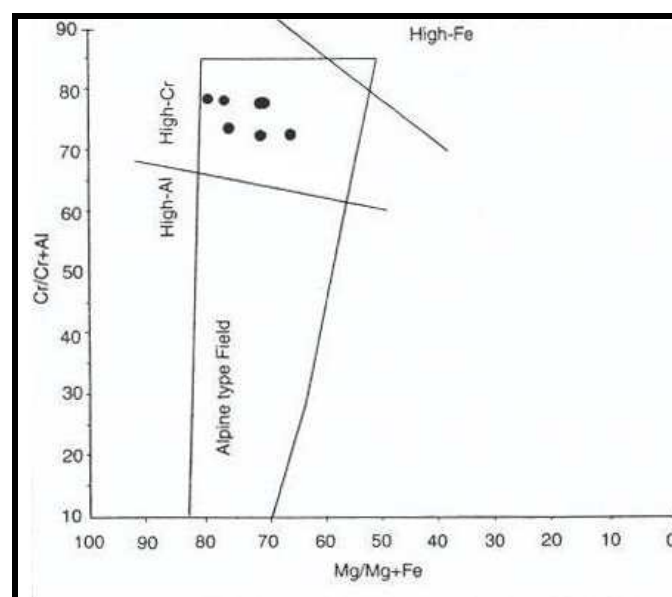
شکل ۱۵ ترسیم نتایج آنالیزهای شیمیایی ذخایر معدنی کرومیت چاه‌یابو و چشمه‌پلنگ در نمودار نسبت \text{Cr}/\text{Cr} + \text{Al} نسبت به \text{Mg}/\text{Mg} + \text{Fe}^{2+} .
