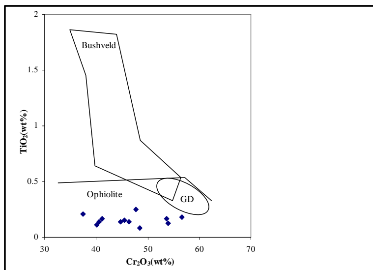
شکل ۱۶ نتایج آنالیزهای شیمیایی ذخایر معدنی کرومیت چاه یابو و چشمه پلنگ در نمودار Cr_2O_3 نسبت به TiO_2 .
