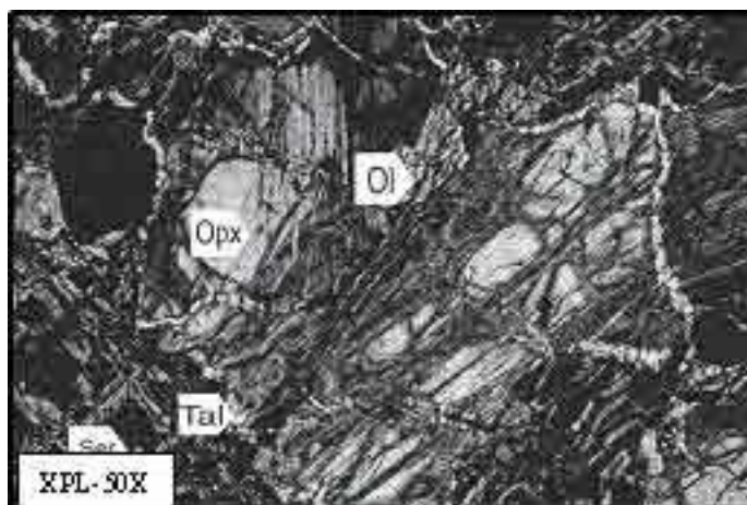
شکل ۳ تصویر میکروسکوپی نور عبوری از هارزبورژیت منطقه ی چشمه پلنگ با بافت پورفیروبلاست (Tal=Talc, Ol= Olivine, Opx= Orthopyroxene, Ser= Serpentine)
