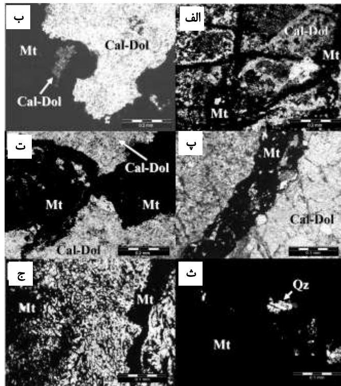
شکل ۳ انواع بافت‌های جانشین در سنگ میزبان در نور قطبشی (PPL). (الف): جانشینی در راستای سطوح لوزی رخ دولومیت-کلسیت، (ب): بافت خوردگی و جزایر بازماندی دولومیت-کلسیت، (پ): مرزهای شکستگی غیر قابل جور شدن (نامتقارن)، (ت): پهن شدگی رگه‌ها در محل شکستگی‌ها، (ث): جزیره‌های جانشین نشده مقاوم کوارتز (Qz) در زمینه مگنتیت، و (ج): رشد تداخلی نامنظم و کرم مانند.
