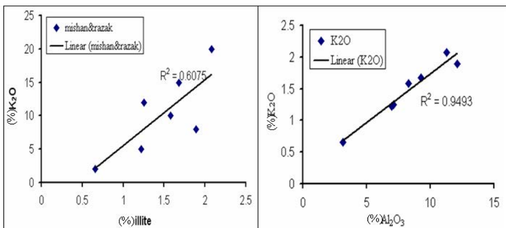
شکل ۹ همبستگی بین ایلیت و K 2 O (٪) نمونه های سازند رازک و میشان.
