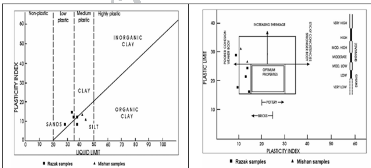
شکل ۷ نمودار کارپذیری نمونه‌های برداشت شده از دو سازند رازک و میشان [۱۹].
