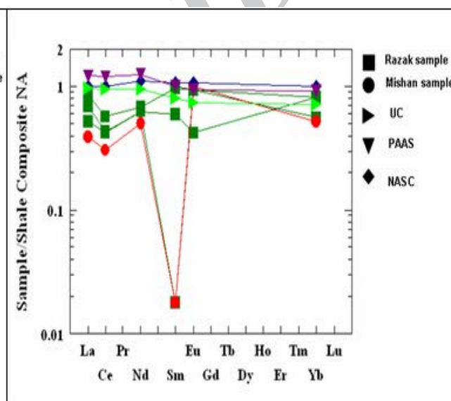
شکل ۴ الگوی توزیع فراوانی REE نمونه‌های رازک و میشان و نمونه‌های استاندارد UC, PAAS, NASC به شیل آمریکا.
