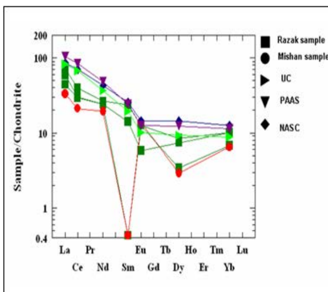
شکل ۵ الگوی توزیع فراوانی REE نمونه‌های رازک و میشان و نمونه‌های استاندارد UC, PAAS, NASC به کندی.
