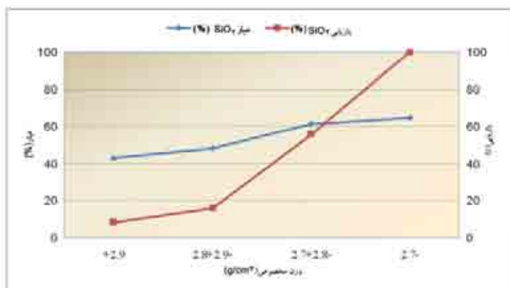
شکل ۹ عیار و بازیابی \text{SiO}_2 محصول نامغناطیسی نسبت به چگالی‌های مختلف. عیار \text{SiO}_2 در آزمون با مایع سنگین با چگالی 2/9 + به 41\% کاهش یافته است.
