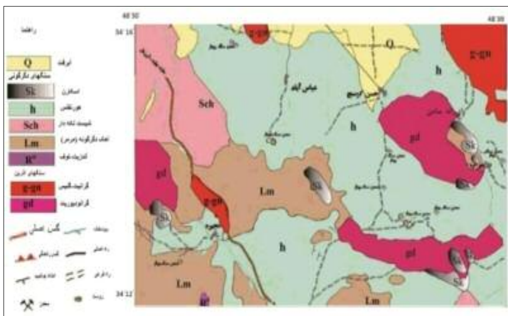
شکل ۱ نقشه زمین‌شناسی و موقعیت هاله‌های دگرگون منطقه‌ی مورد بررسی، اقتباس از نقشه‌ی ۱:۱۰۰۰۰۰ مایلی [۱].
