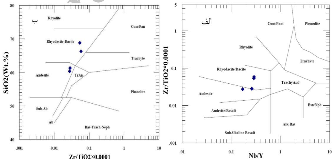
شکل ۵ موقعیت نمونه‌ها در نمودار الف: Nb/Y نسبت به Zr/TiO_2 [۱۲] ب: نمودار Zr/TiO_2 نسبت به SiO_2 [۱۲].
