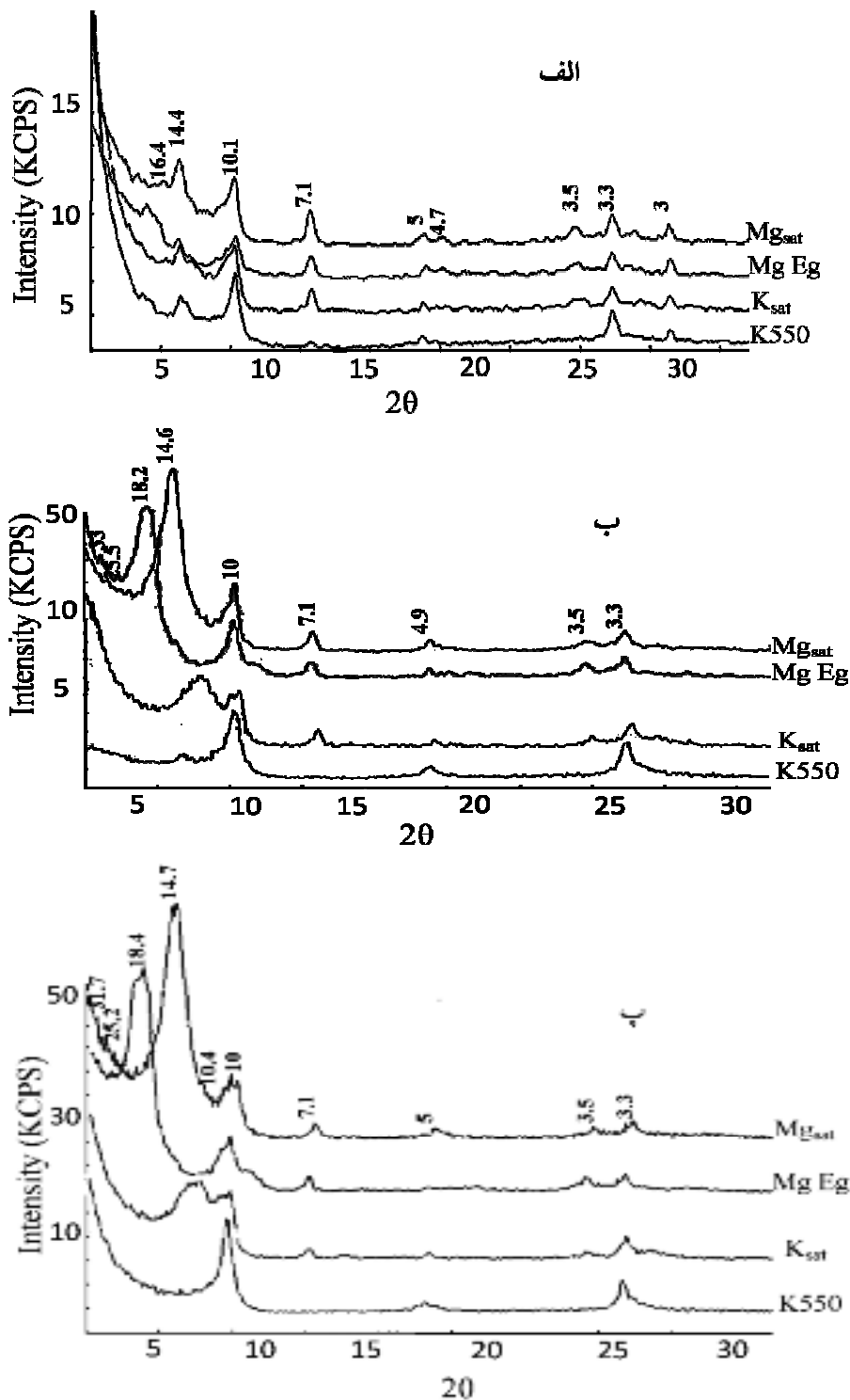
شکل ۳ پراش‌نگاشت‌های رس خاکرخ گرانیتی (Gr1. الف) افق A1، ب) افق Bw، پ) افق C. نمونه‌ی اشباع با منیزیم، Mg Eg نمونه‌ی اشباع با اتیلن گلیکول، Ksat و K550 به‌ترتیب، نمونه‌های اشباع با پتاسیم و دمای ۵۵۰ درجه سانتی‌گراد.
