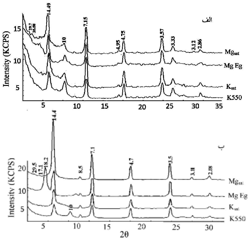
شکل ۲ پراش‌نگاشت‌های رس در خاکرخ فوق‌بازی Ub2 (الف افق A، ب افق Cry، Mgsat نمونه اشباع با منیزیم، Mg Eg نمونه اشباع با منیزیم و اتیلن گلیکول، K 550 و K sat به‌ترتیب نمونه‌های اشباع با پتاسیم و حرارت ۵۵۰ درجه سانتی‌گراد، اعداد بر روی قله پراش‌نگاشت‌ها، بر حسب آنگستروم می‌باشند.
