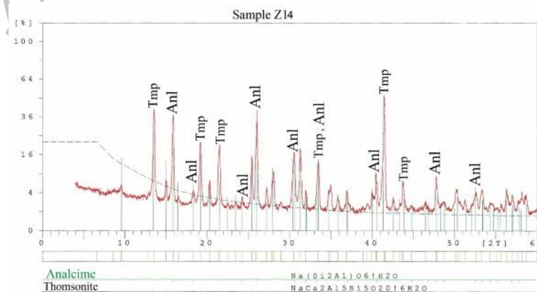
شکل ۳ الگوی پراش پرتو X مربوط به آمیگدال زئولیتی منطقه حرمت که دو فاز آنالسیم (Anl) و تامسونیت (Tmp) در آن قابل تشخیص است. علائم اختصاری از کرتز (۱۹۸۳) است [۸].
