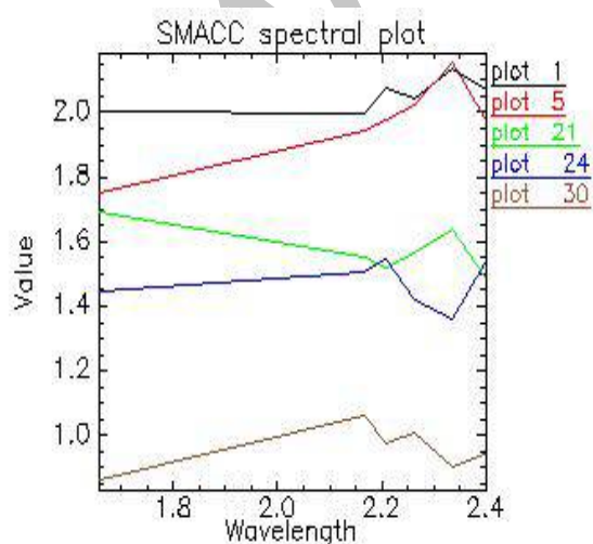
شکل ۳ طیف‌های SMACC حاصل از نامیختگی طیفی تکراری منطقه‌ی جمیله، الف: دسته داده‌های ۹ بانندی؛ ب: دسته داده‌های ۶ بانندی.
