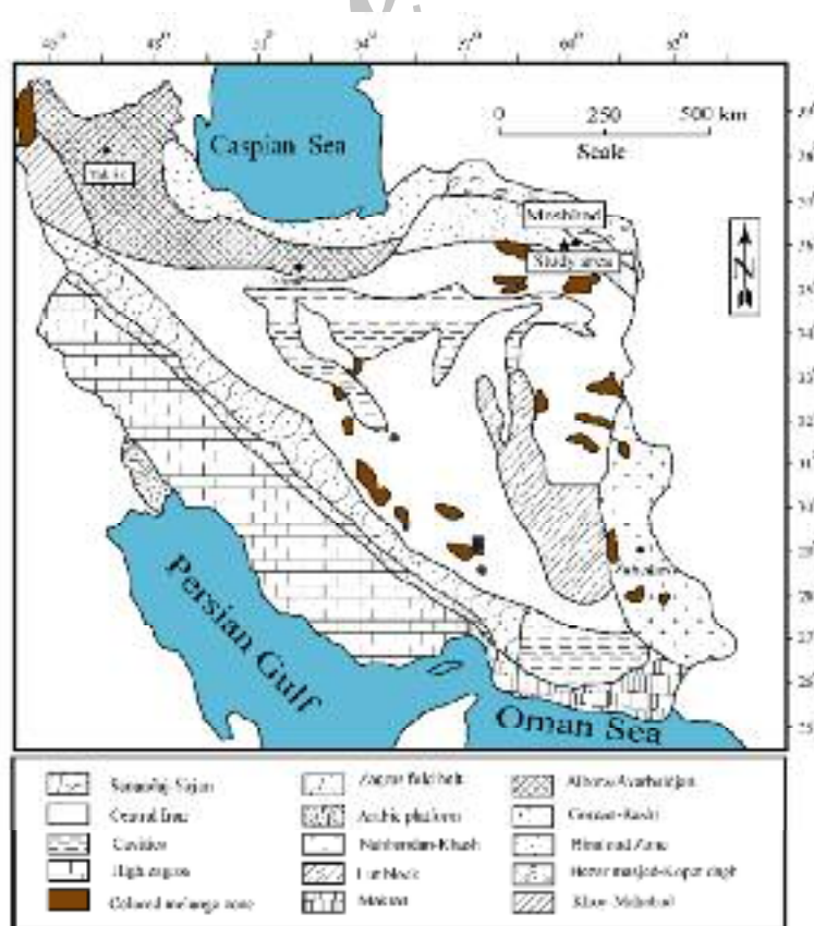
شکل ۱ موقعیت منطقه‌ی مورد بررسی در نقشه‌ی زون‌های ساختاری ایران [۱].
