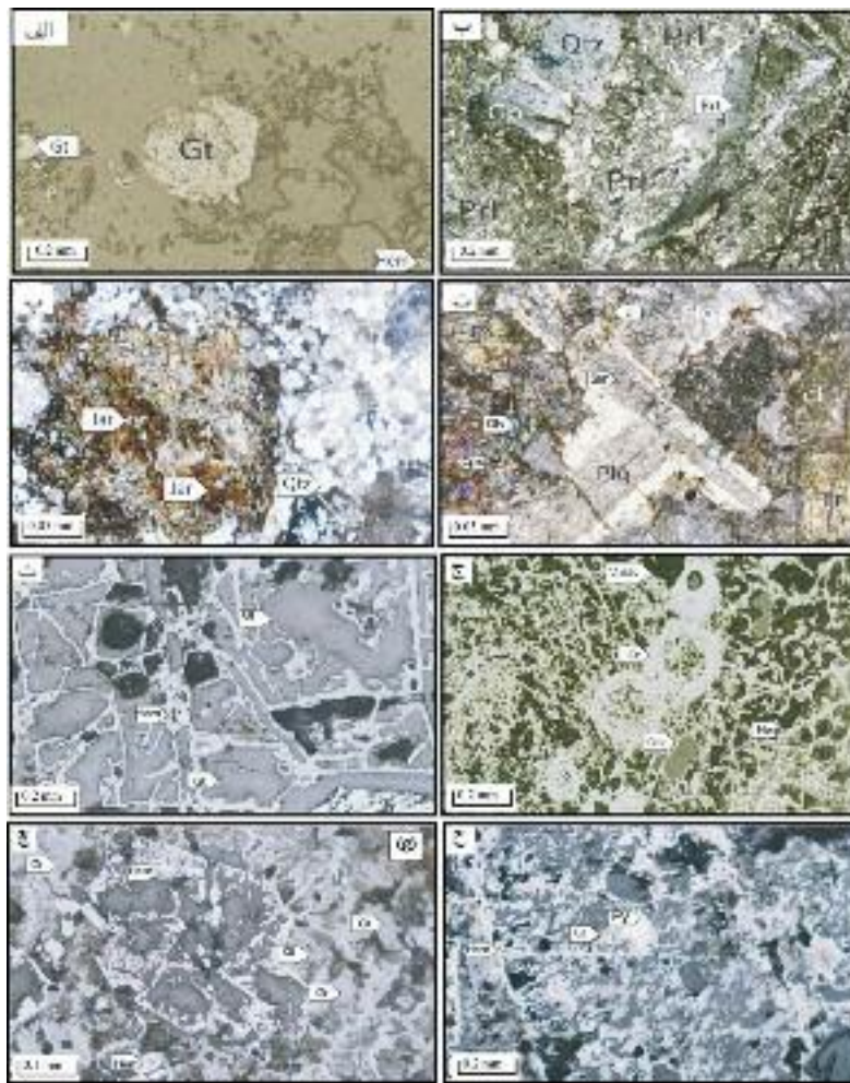
شکل ۶ الف- گوتیت شبه‌ریخت پس بعد از پیریت در ماسه‌سنگ‌های آهن‌دار. نور انعکاسی (PPL). ب- ژپیس، باریت، و پیروفلیت در ماسه‌سنگ آهن‌دار. نور انعکاسی (XPL). پ- جاروسیت به همراه کوارتز در ماسه‌سنگ‌های آهن‌دار. نور انعکاسی (XPL). ت- پلاژیوکلازهای سریسیتی شده و کلریت در دایک‌های منطقه. نور انعکاسی (XPL). ث- هماتیت و گوتیت با بافت اسکلتی که در آن گوتیت در فضای بین دیواره‌های حاصله از هماتیت باقی مانده است. نور انعکاسی. ج- شبه‌ریخت گوتیت پس از پیریت. نور انعکاسی. چ- جانشینی گوتیت به وسیله هماتیت و بافت جانشینی برجای مانده. نور انعکاسی. ح- جانشینی حاشیه‌ای پیریت توسط گوتیت. نور انعکاسی. علائم اختصاری بکار رفته عبارتند از: Py= پیریت، Hem= هماتیت، Lm= لیمونیت، Gt= گوتیت، Qtz= کوارتز، Brt= باریت، Prl= پیروفلیت، Jar= جاروسیت، Plg= پلاژیوکلاز، Cl= کلریت، Ser= سریسیت، Olv= الیون، و Cpx= کلینوپیروکسن.
