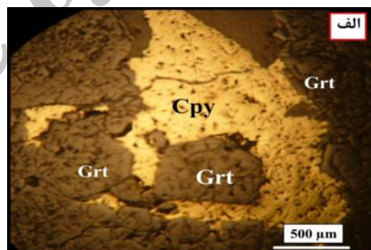
شکل ۴ الف: کالکوپیریت به صورت شکافه پرکن در فضای بین گارنت‌ها ب: کانه‌زایی پیروتیت به صورت افشان و کانه‌زایی اسفالریت به شکل رگچه‌ای در مرمرها (Cpy: کالکوپیریت؛ Grt: گارنت؛ Sp: اسفالریت).
