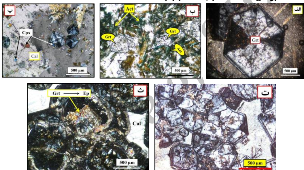
شکل ۳ الف: زون بندی نوسانی گارنت‌های ناهمسانگرد در اسکارن‌های منطقه خوت. ب: جانشینی گارنت توسط اکتینولیت در مرحله متاسوماتیسم پسرونده. پ: وجود ادخال‌های کلینوپیروکسن در گارنت‌های ناهمسانگرد. ت: بافت دانه‌ای در گارنت‌های ناهمسانگرد در مرحله متاسوماتیسم پیشرونده. ث: گارنت‌های همسانگرد خود شکل با بافت گرانولار در اسکارن پیشرونده و دگرسانی مرکز آن به اپیدوت و کلریت. (Grt: گارنت؛ Ep: اپیدوت؛ Act: اکتینولیت).
