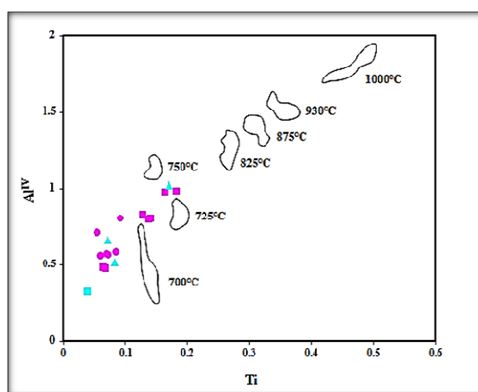
شکل ۷ محاسبه‌ی تقریبی دمای تشکیل آمفیبول‌های توده‌های گرانیتوئیدی نشوه و سلیجراد براساس روش هلز [۲۰].
