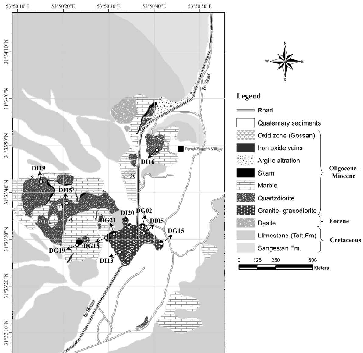
شکل ۱ نقشه زمین‌شناختی منطقه دره زرشک و موقعیت اسکارن‌ها و نمونه‌ها روی آن.
