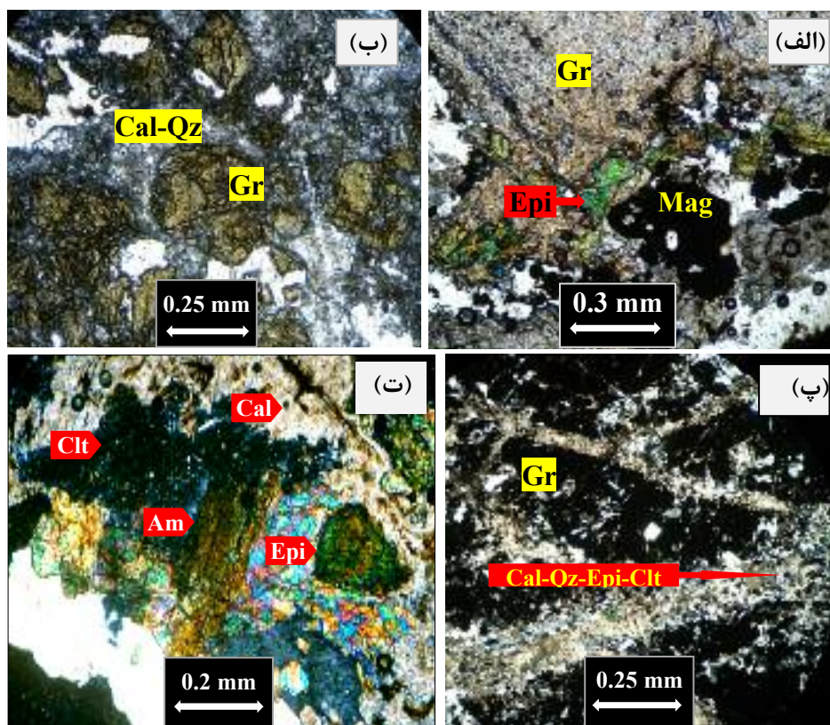
شکل ۴ (الف) تشکیل مگنتیت و اپیدوت از راه جاننشینی گارنت (PPL)؛ (ب) خردشدگی و سیمانی شدن گارنت به وسیله‌ی کوارتز و کلسیت در مرحله‌ی دگرسانی قهقرایی (PPL)؛ (پ) قطع اسکارن پیشرونده با رگچه‌های اسکارن قهقرایی (XPL)؛ (ت) تشکیل کلریت از راه جاننشینی اپیدوت و آمفیبول در مرحله‌ی دگرسانی پسرونده (XPL)؛ (د) علایم اختصاری: Gr: گارنت، Mag: مگنتیت، Epi: اپیدوت، Cal: کلسیت، Qz: کوارتز، Clt: کلریت، Am: آمفیبول.
