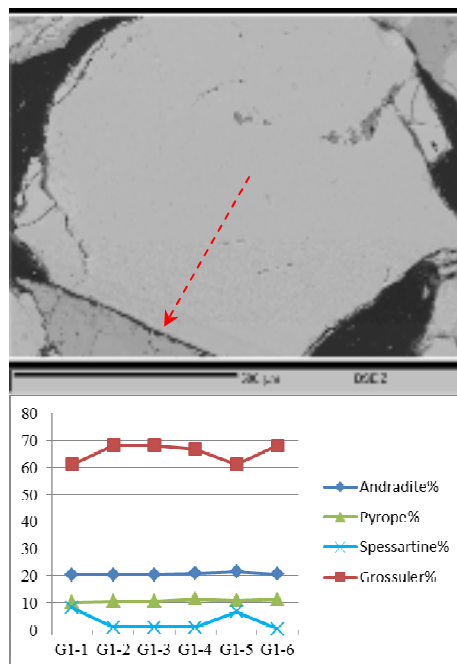
شکل ۱۱ تصویر BSE کانی گارنت و نمودار درصد تغییرات نوع گارنت در راستای پیمایش (مرکز به حاشیه) ریزکاونده‌ی الکترونی (داده‌های پیمایش ۱ در جدول ۲).
