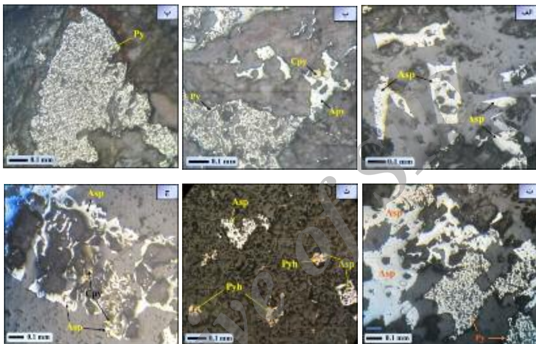
شکل ۹ تصاویر میکروسکوپی از کانی‌سازی‌های مختلف در منطقه‌ی پی‌جوئی فیروزکوه (تور PPL). (پیریت: Py، آرسنوپیریت: Asp، کالکوپیریت: Cpy، پیروتیت: Phy) الف) کانی آرسنوپیریت با اشکال مختلف لوزی و مثلثی. ب) پاراژنز پیریت- آرسنوپیریت- کالکوپیریت. پ) کانی‌سازی پیریت (ت) پاراژنز پیریت- آرسنوپیریت (ث) پاراژنز آرسنوپیریت- پیروتیت (ج) تشکیل کالکوپیریت روی آرسنوپیریت.
