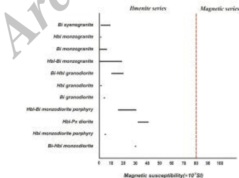
شکل ۳ پذیرفتاری مغناطیسی توده‌های نفوذی منطقه پی‌جوئی فیروزکوه. (همه‌ی نمونه‌ها در محدوده‌ی سری ایلمنیتی جای می‌گیرند).
