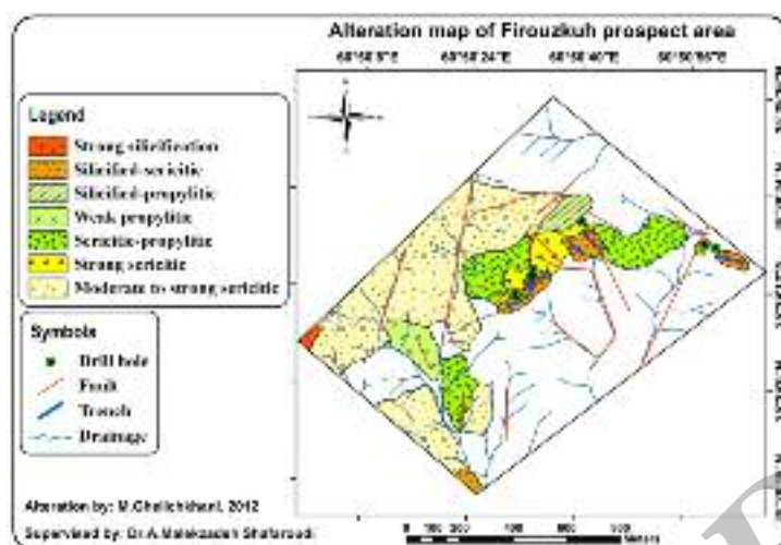
شکل ۸ نقشه‌ی دگرسانی منطقه‌ی پی‌جوئی فیروزکوه همراه با موقعیت گمانه‌ها و ترانسه‌ها.
