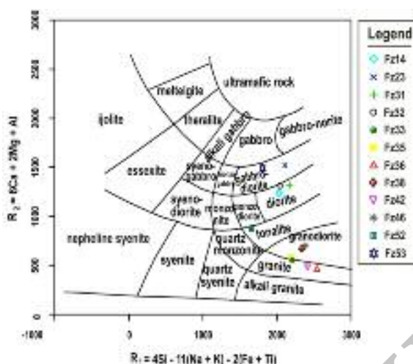
شکل ۴ نمودار نامگذاری سنگ‌های آذرین درونی با استفاده از نسبت کاتیون‌ها [۱۱]. نمونه‌های فیروزکوه در محدوده گرانیت، گرانودیوریت، دیوریت، تونالیت و گابرودیوریت قرار می‌گیرند.
