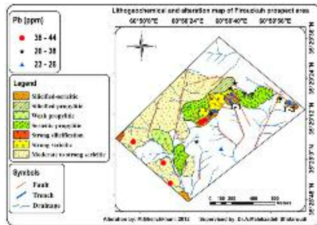
شکل ۱۴ نقشه ژئوشیمی عنصر سرب منطقه‌ی پی جوئی فیروزکوه.
