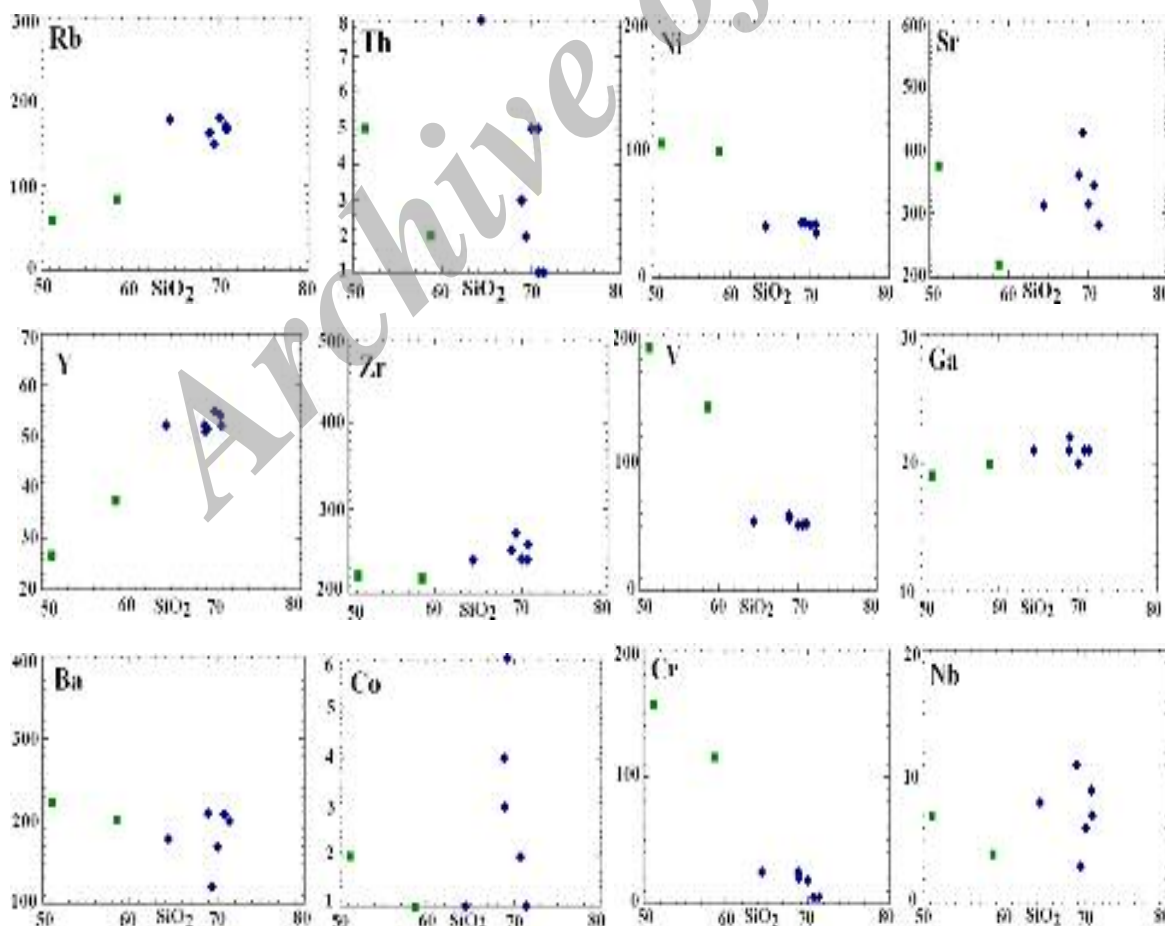
شکل ۹ نمودارهای تغییرات اکسیدهای عناصر فرعی (بر حسب ppm) نسبت به اکسید سیلیسیم [۹].
