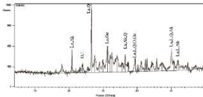
شکل ۱۱ پراش نگاشت حاصل از آنالیز پراش پرتو ایکس (XRD)، نمونه‌ی آجر MH-6. راهنما: کوارتز: Q لارنیت: La آکرمانیت: Ak ژلنیت: Ge ارتوکلاز: O
