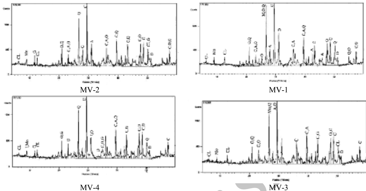
راهنما: کوآرتز: Q؛ مونت مویلونیت: Mn؛ مسکویت: Mo؛ دولومیت: D؛ ارتوکلاز: O؛ ایلیت: I؛ کلریت: Cl؛ آلبیت: A. ادامه شکل ۵ پراش نگاشت‌های پرتو ایکس (XRD) ۴ نمونه‌ی برداشت شده از سازند میشان.
